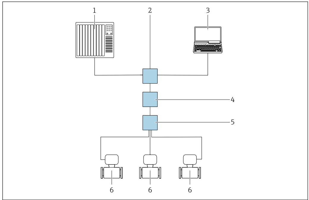
48 Opzioni per il funzionamento a distanza tramite il protocollo Modbus TCP su Ethernet-APL (attivo)
