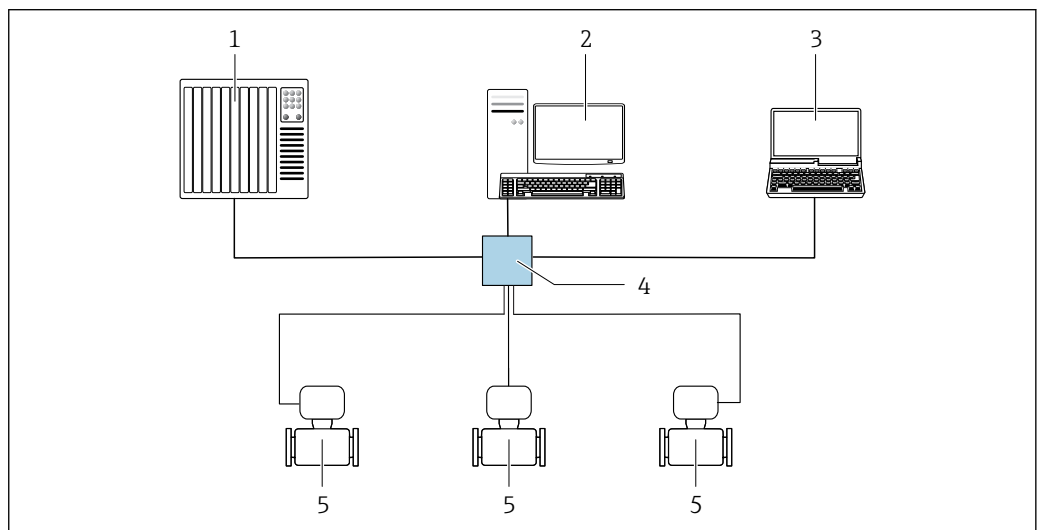
49 Opzioni per il funzionamento a distanza tramite Modbus TCP su Ethernet - 100 Mbit/s: topologia a stella
