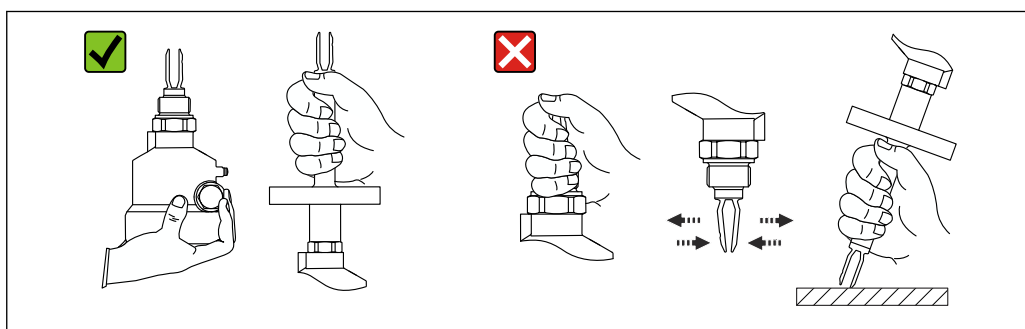
3 Manejo del equipo durante el transporte
