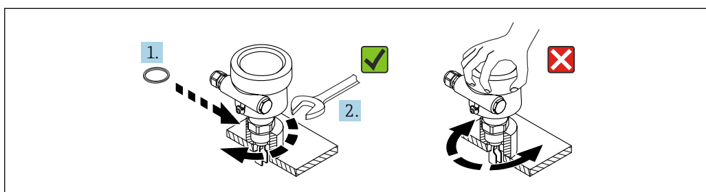
15 Enroscado del equipo
