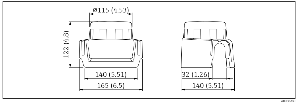
23 Tapa de protección ambiental para caja de compartimento único de aluminio. Unidad de medida mm (in)
