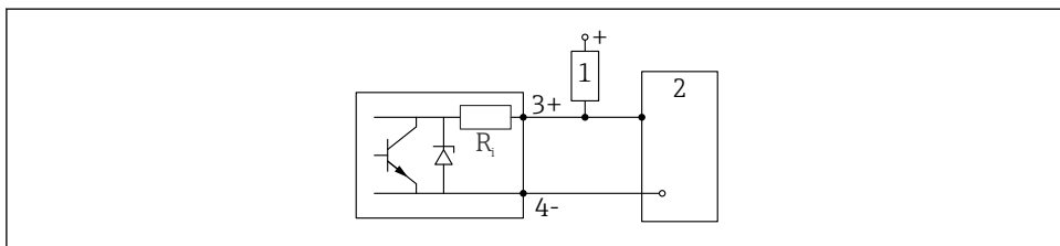
6 Esempio di connessione per l'ingresso digitale
