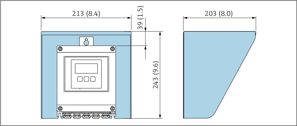
19 Tapa de protección ambiental para Proline 500, digital; unidad mm (in)
