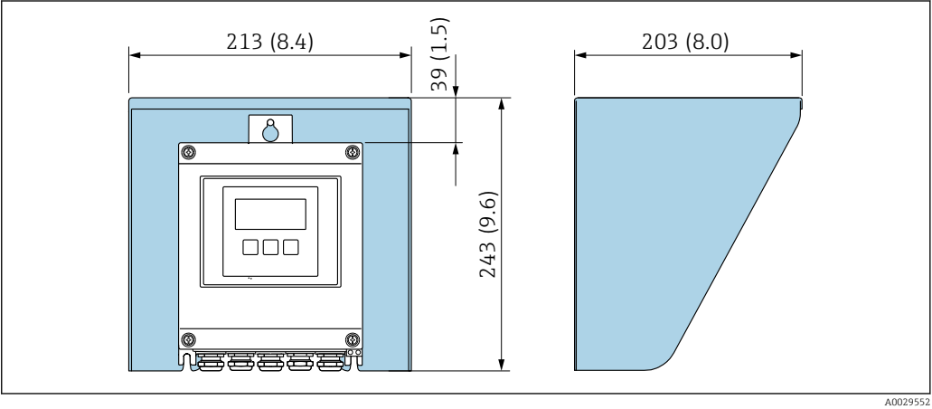
27 Tapa de protección ambiental para Proline 500, digital; unidad mm (in)
