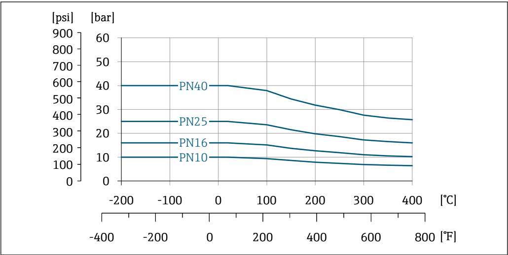
16 Materiale della connessione flangiata: acciaio inox, certificazioni multiple, 1.4404/F316/F316L
