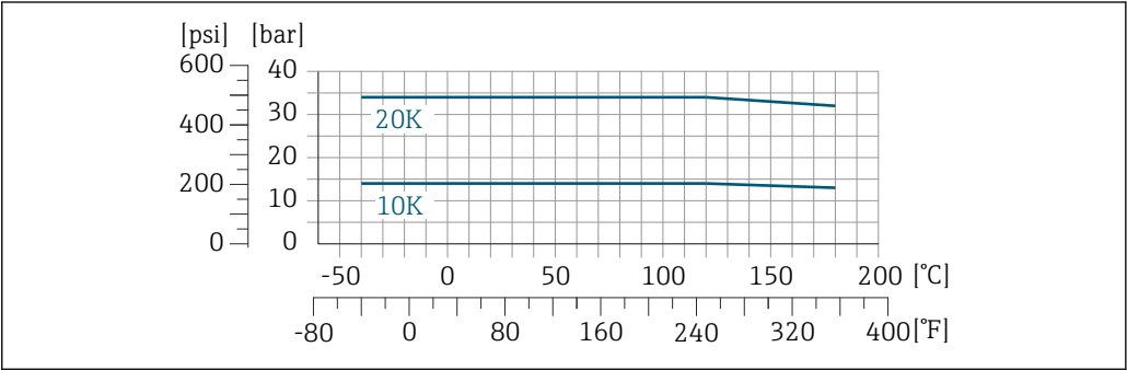
18 Materiale della connessione flangiata: acciaio inox, certificazioni multiple, 1.4404/F316/F316L
