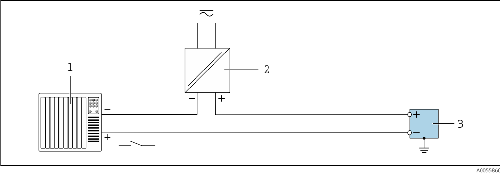
19 Exemple de raccordement pour l'entrée état 1 Système d'automatisation avec sortie tout ou rien passive p. ex. API) 2 Alimentation électrique 3 Transmetteur avec entrée d'état
