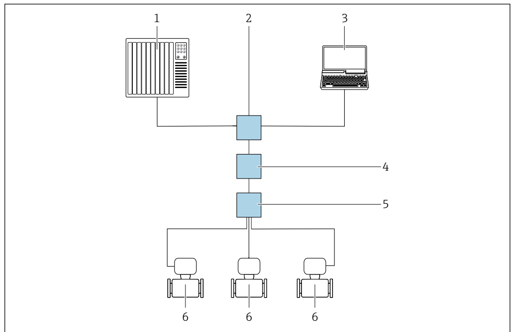
25 Options de configuration à distance via Modbus TCP sur protocole Ethernet-APL (active)
