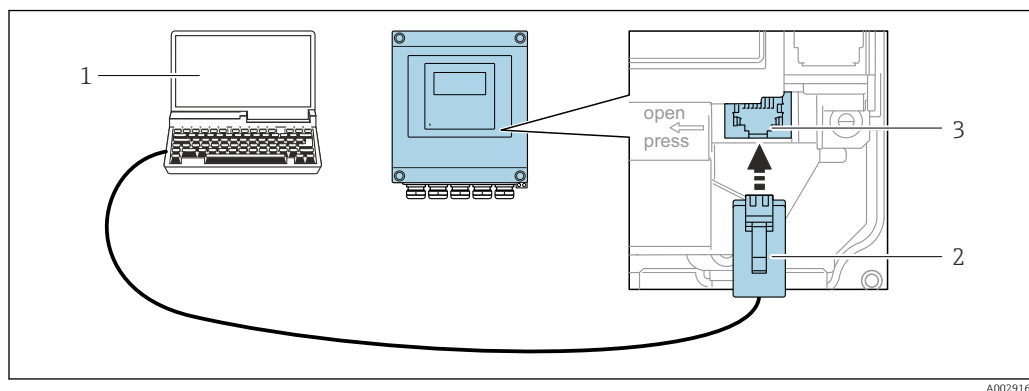
29 Подключение через сервисный интерфейс (CDI-RJ45)
