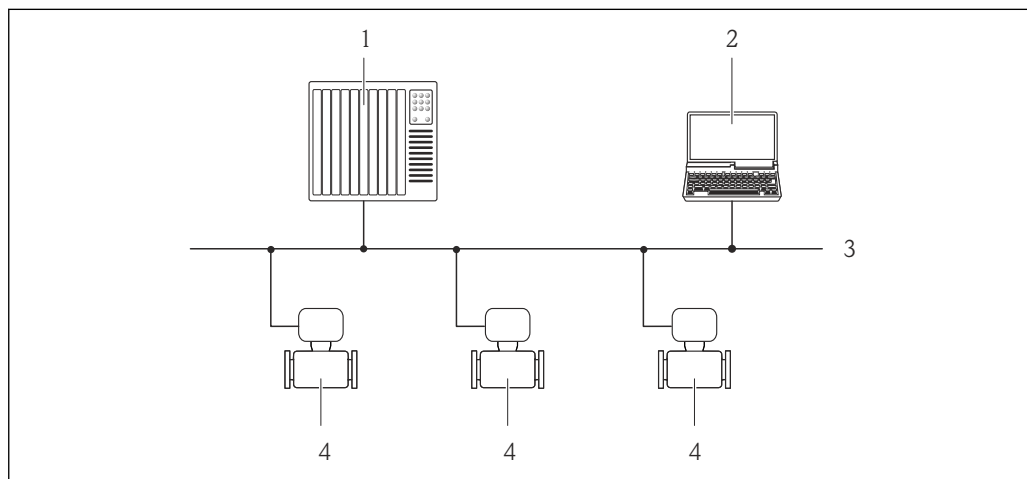
28 Варианты дистанционного управления через сеть PROFIBUS DP
