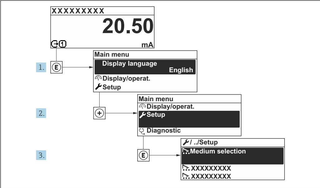
32 Переход к меню "Настройка" на примере местного дисплея
