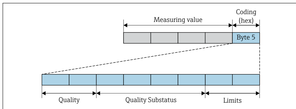
36 Структура байта кодирования
