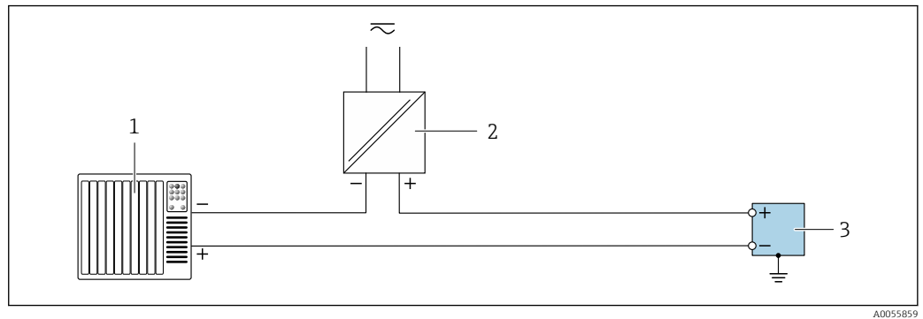
21 Пример подключения для релейного выхода
