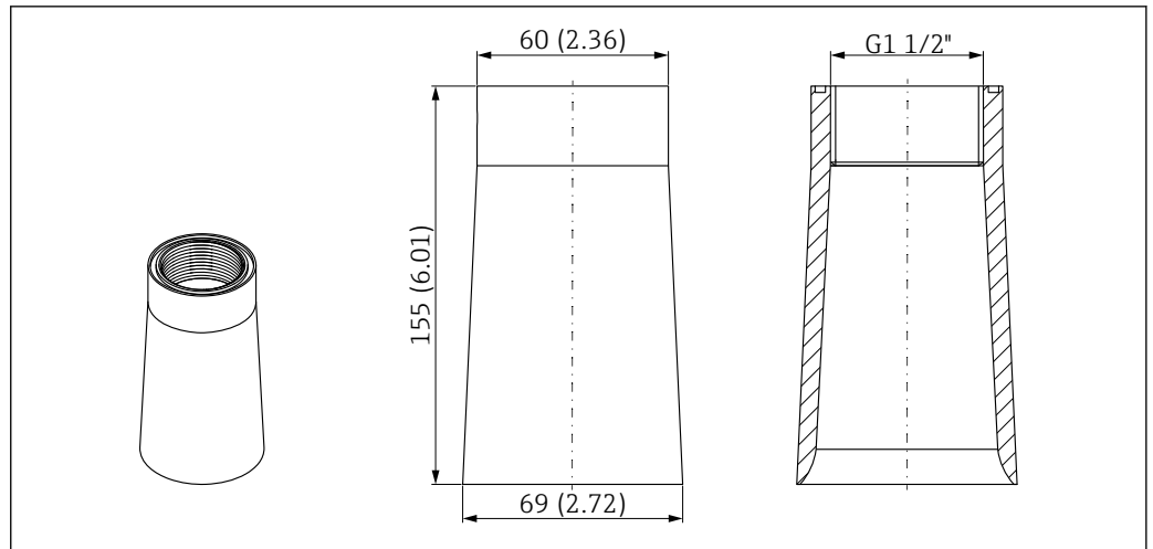
32 Dimensions du tube de protection antidébordement 40 mm (1,5 in). Unité de mesure mm (in)
