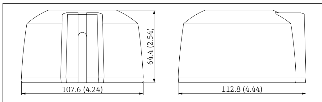
27 Dimensions pour capot de protection avec entrée de câble par le côté. Unité de mesure mm (in)
