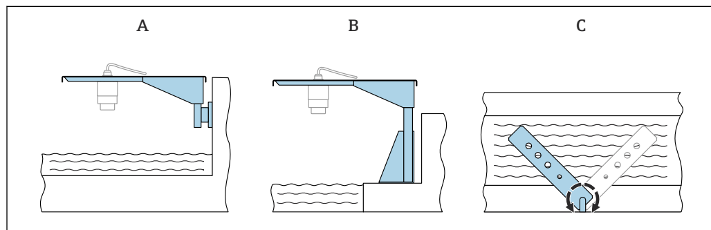
8 Montage avec bras de montage, avec pivot
