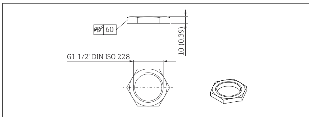
28 Dimensions de l'écrou de fixation. Unité de mesure mm (in)
