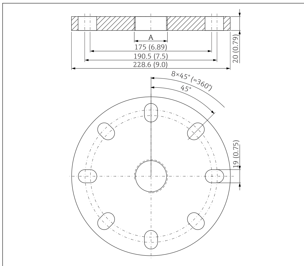
55 Dimensions de la bride UNI 4"/DN100/100. Unité de mesure mm (in)
