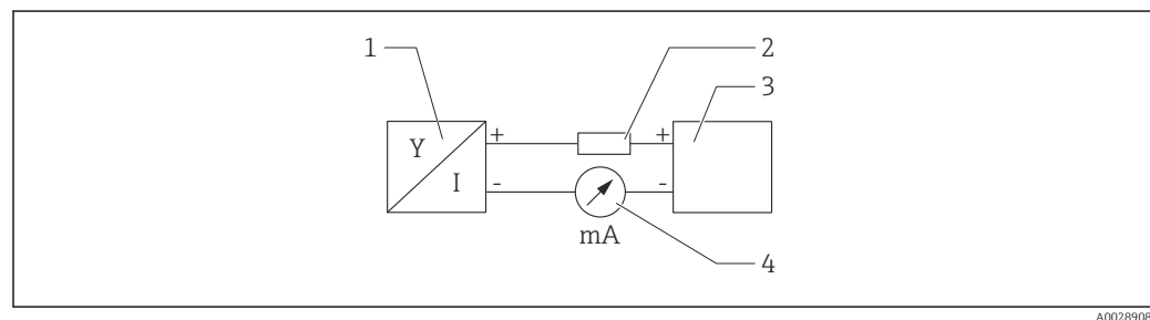
11 Schéma de principe de la connexion HART
