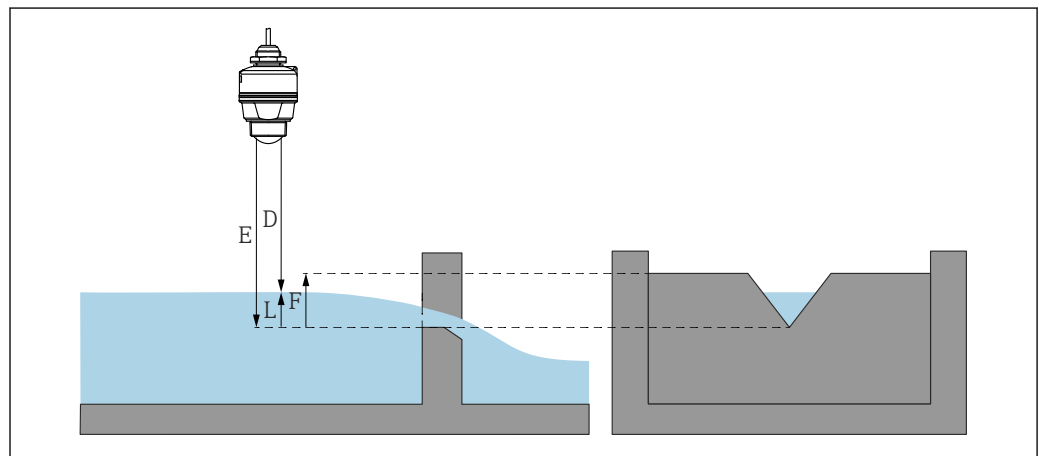
24 Exemple : déversoir en V
