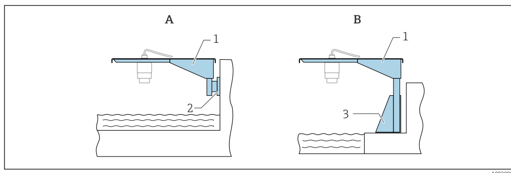
39 Type de montage raccord process à l'entrée de câble capteur
