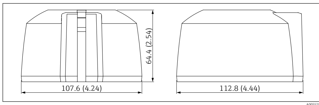
26 Dimensions pour capot de protection G1/NPT1, entrée de câble par le haut. Unité de mesure mm (in)
