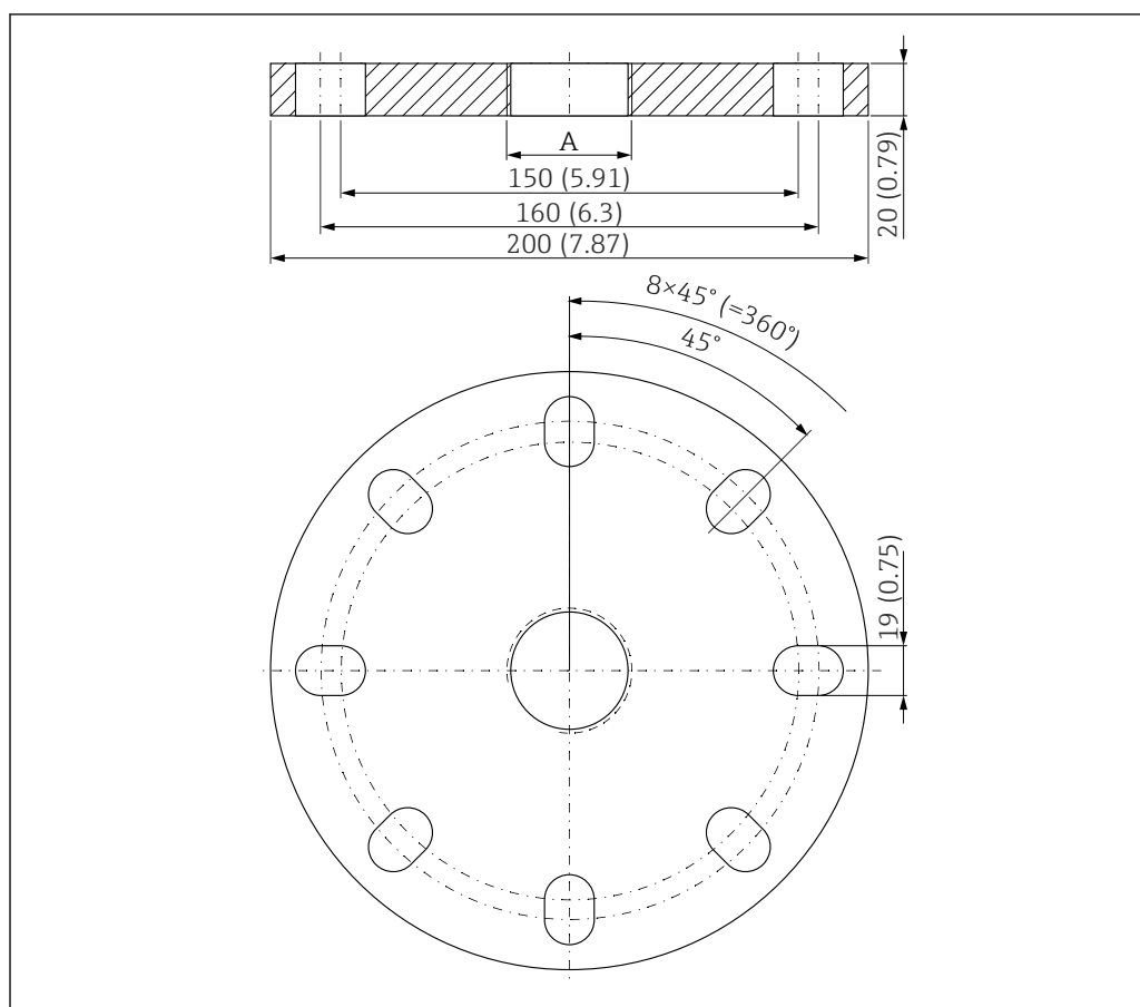
54 Dimensions de la bride UNI 3"/DN80/80. Unité de mesure mm (in)
