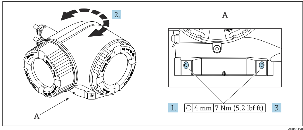
图 15 防爆型外壳
