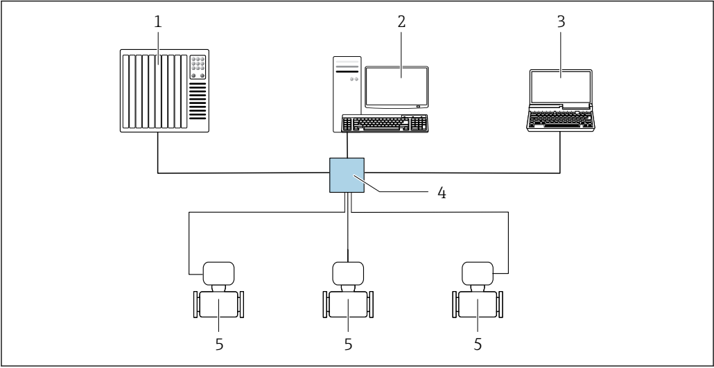
图 30 通过 Modbus TCP + Ethernet 进行远程操作 - 100 Mbit/s: 星形拓扑结构
