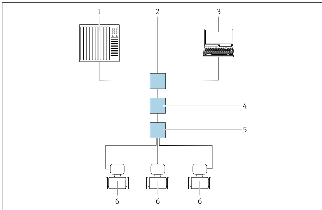
图 29 通过 Modbus TCP + Ethernet-APL 通信进行远程操作（有源信号）
