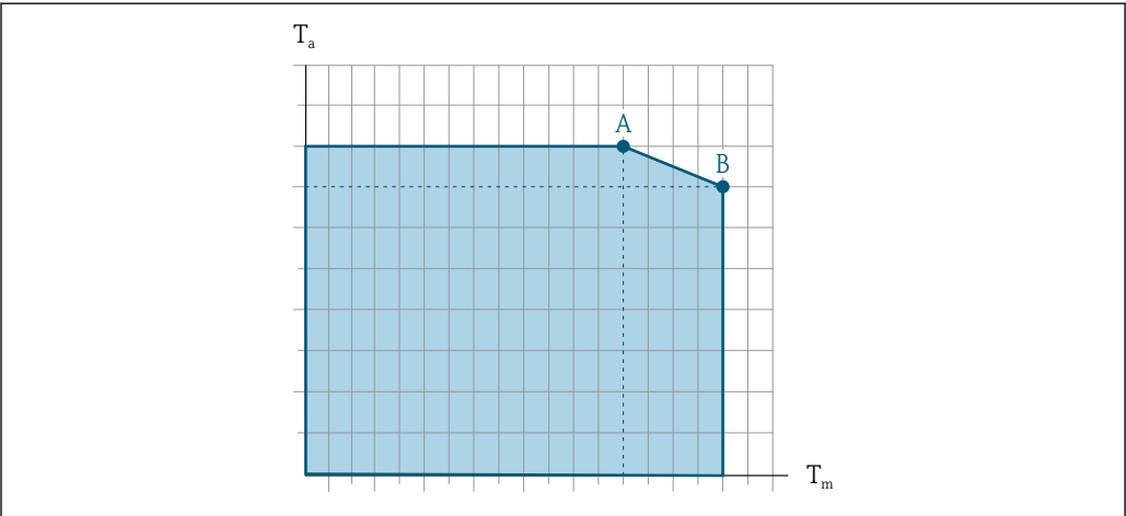
图 33 示例图，具体数值见下表。 T a 环境温度 T m 介质温度 A 介质温度 T m 越高 (T a max = 60 °C (140 °F)时)，所需的环境温度 T a 越低 B 传感器最高允许介质温度 T m 对应的最高允许环境温度 T a
