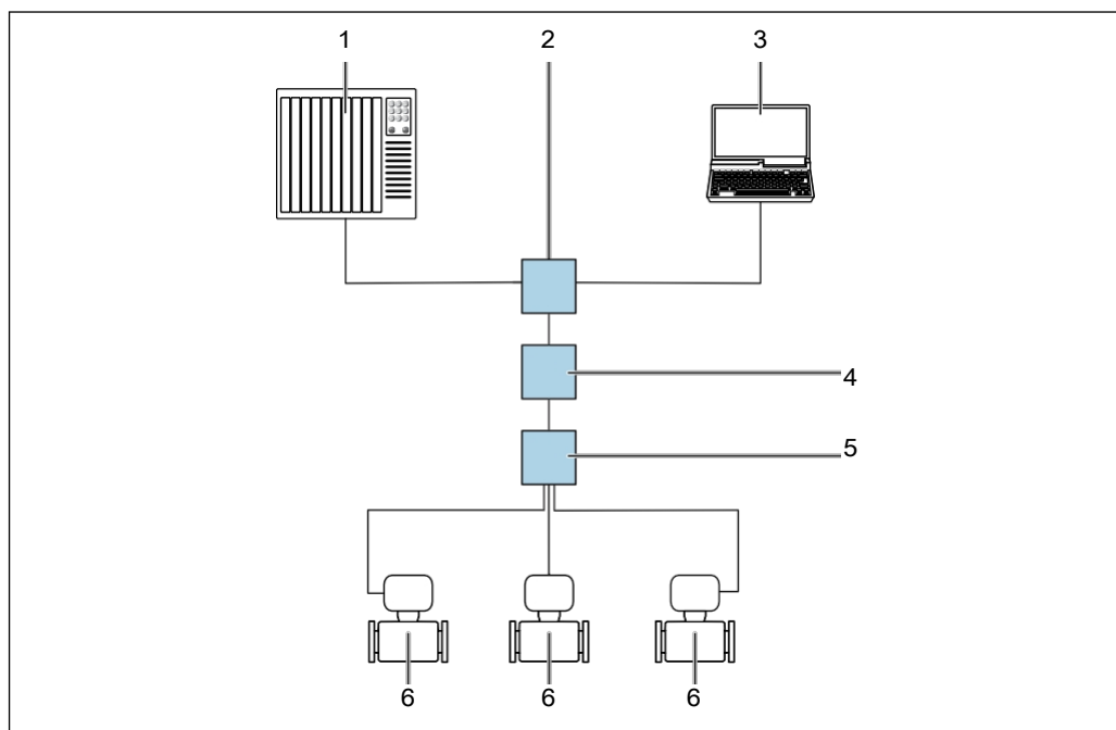
□ 69 Možnosti dálkového ovládání prostřednictvím sítě APL
