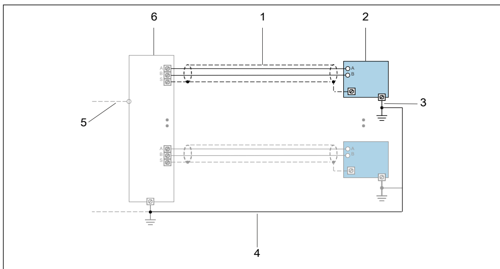
□ 13 Příklad připojení pro Modbus s TCP-APL
