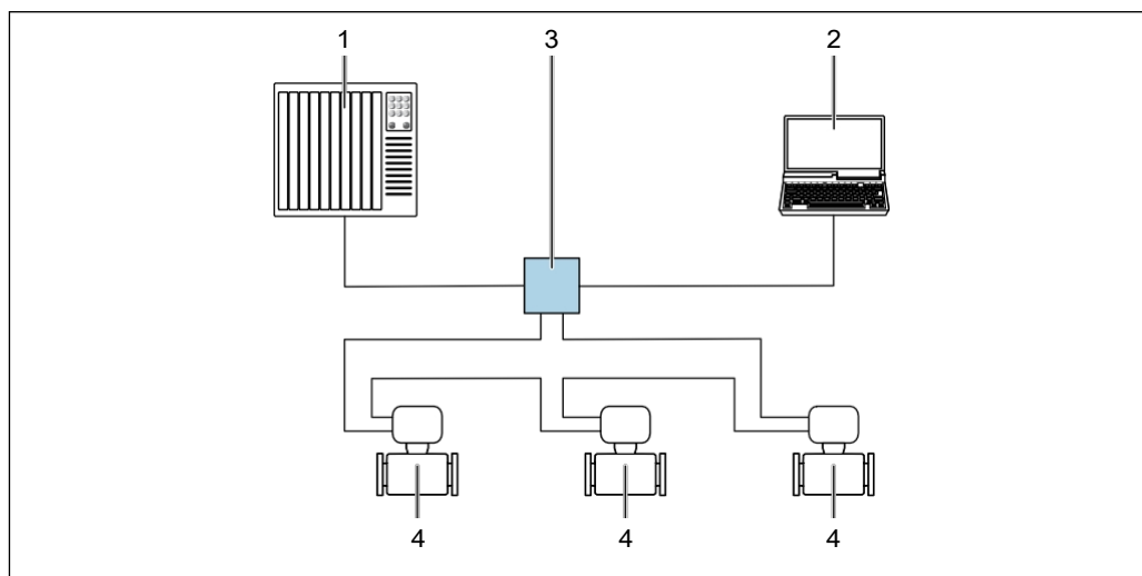
□ 68 Možnosti vzdáleného provozu přes síť PROFINET: kruhová topologie
