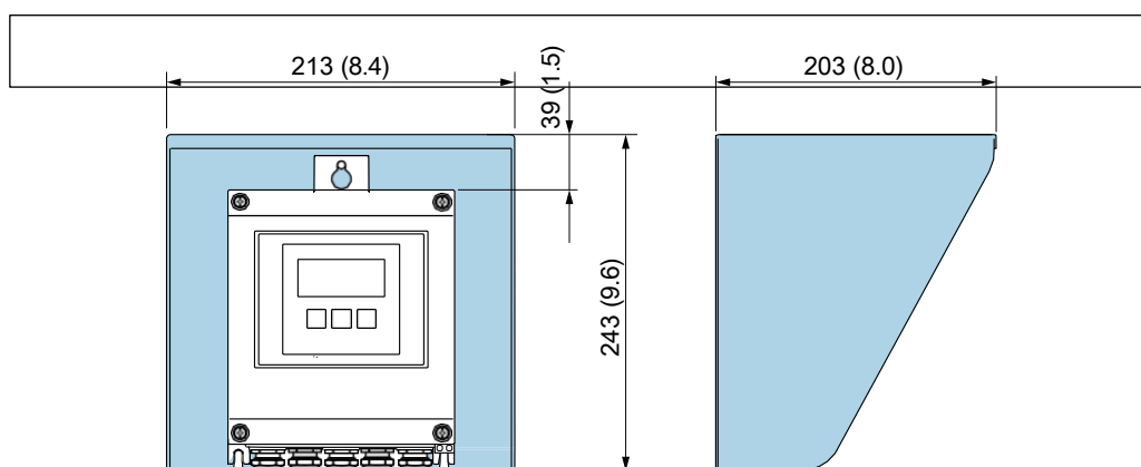
□ 45 Kryt proti povětrnostním vlivům pro Proline 500 - digitální; technická jednotka mm (in)
