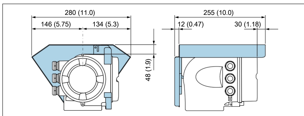
□ 46 Kryt proti povětrnostním vlivům pro Proline 500; technická jednotka mm (in)
