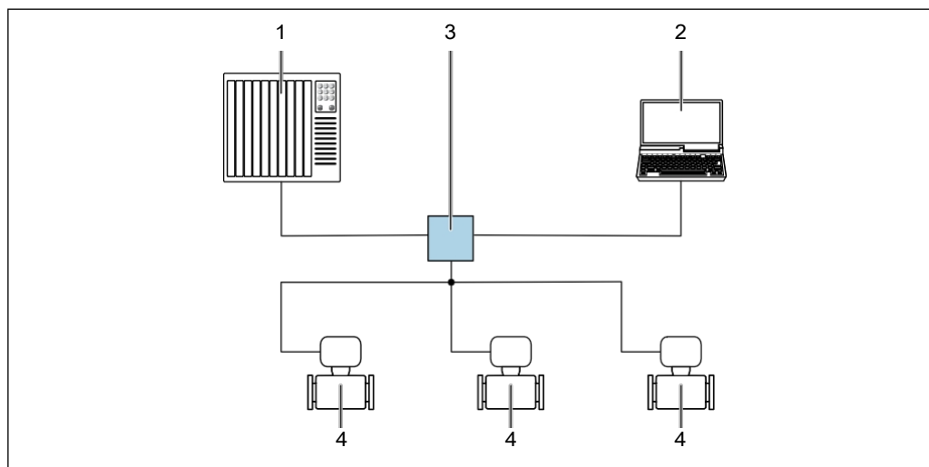
□ 67 Možnosti dálkového ovládání prostřednictvím sítě PROFINET: hvězdicová topologie
