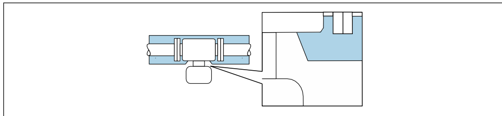
□ 42 Tepelná izolace s odkrytým prodlouženým hrdlem
