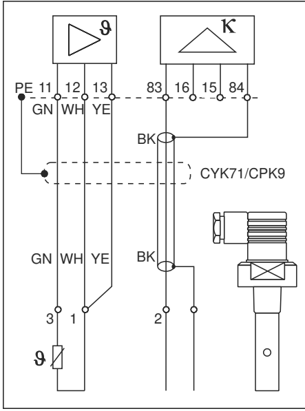
7 İletken sensörlerin bağlantısı
