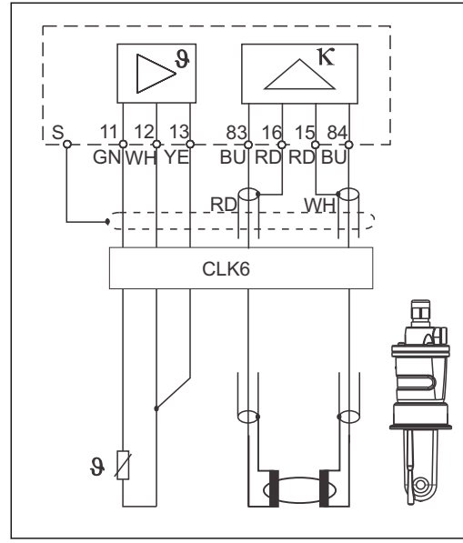
8 Endüktif sensörlerin bağlantısı
