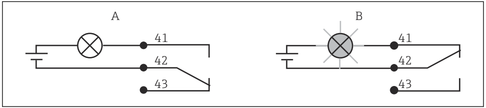
9 Tavsiye edilen arıza emniyetli alarm bağlantı anahtarı
