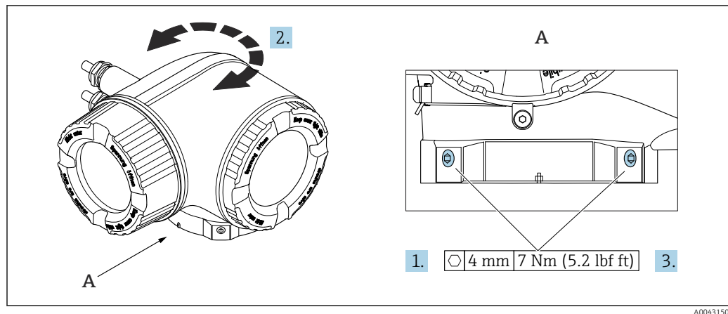
11 Boîtier Ex
