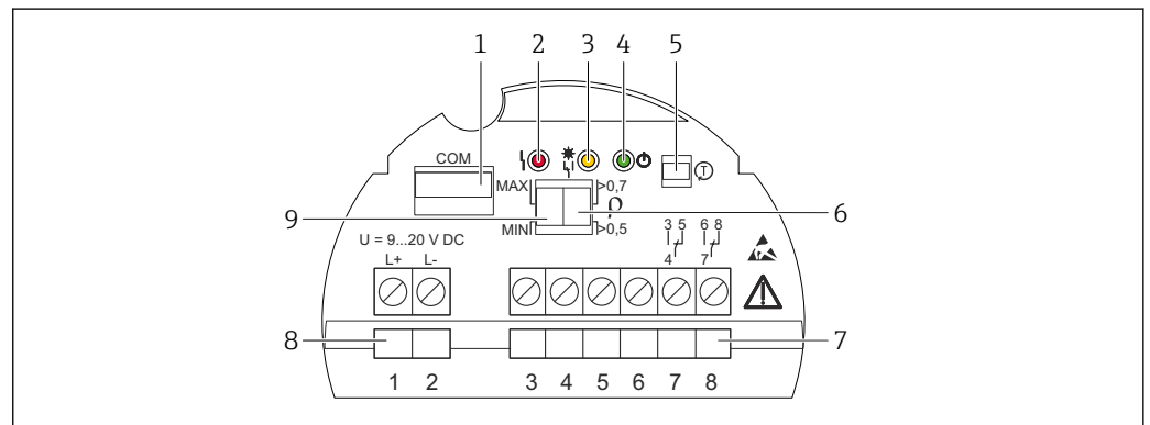
Fig. 33 Ejemplo de módulo del sistema electrónico FEL64DC
