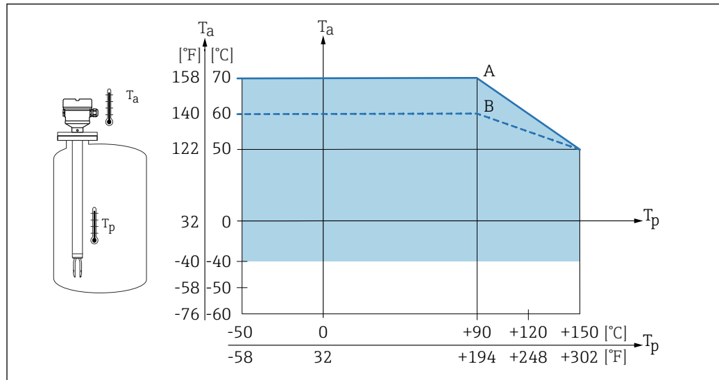
52 Temperatura ambiente admisible T_a en la caja en función de la temperatura de proceso T_p en el depósito:
