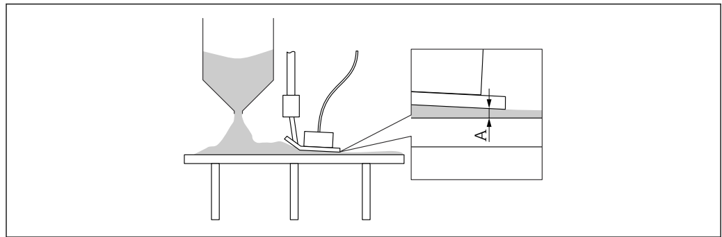
図 11 コンベヤーベルトの上への丸型センサの設置
