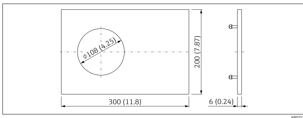
図 33 バッフルプレート、1.4301、センサ切り欠き \varnothing 108 mm (4.25 in)。測定単位 mm (in)
