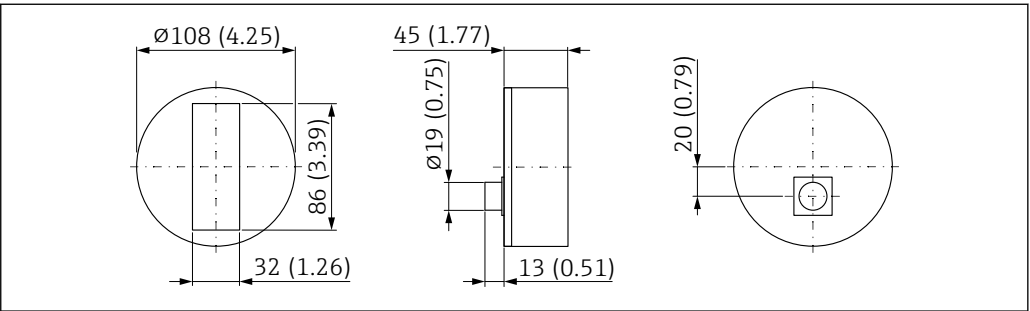
図 18 丸型センサ（ショート）の寸法。測定単位 mm (in)
