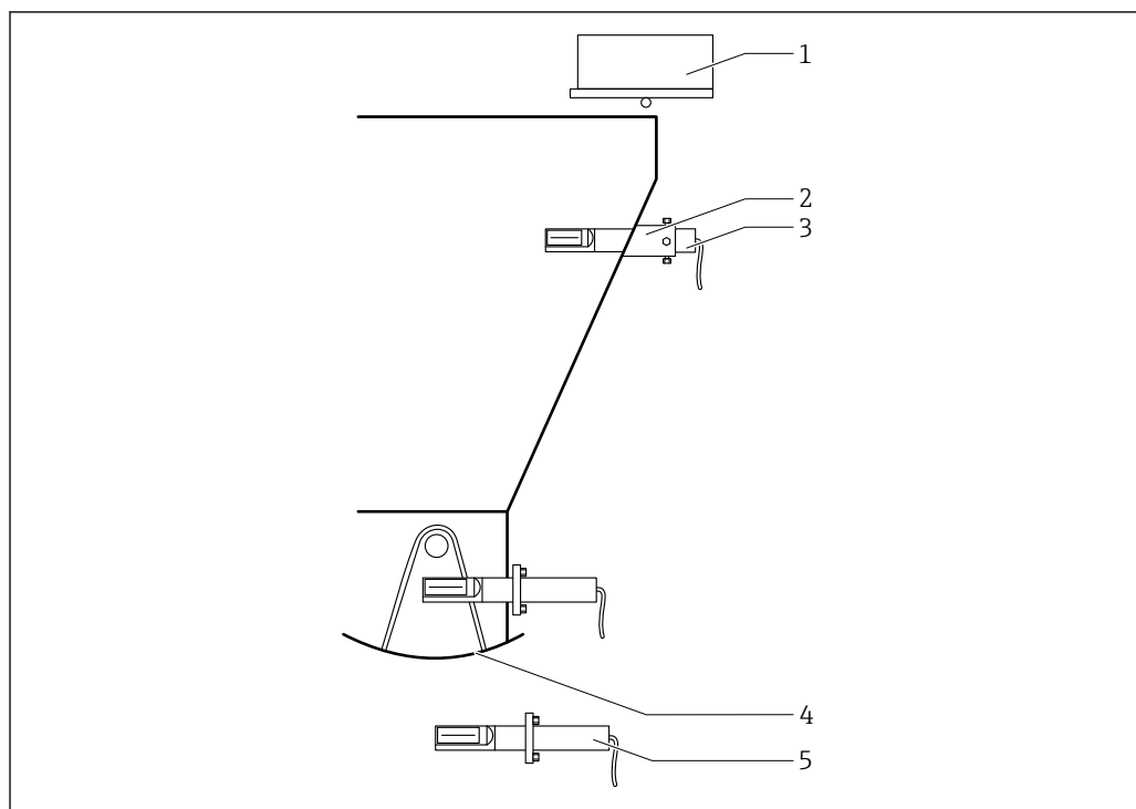
図 15 サイロへのロッドセンサの設置
