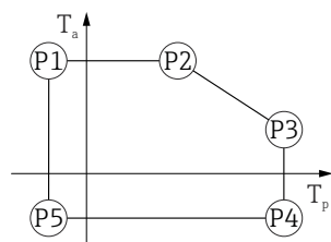
49 316L 外壳，卫生型；过程温度范围：-20 ... +200 °C (-4 ... +392 °F)
