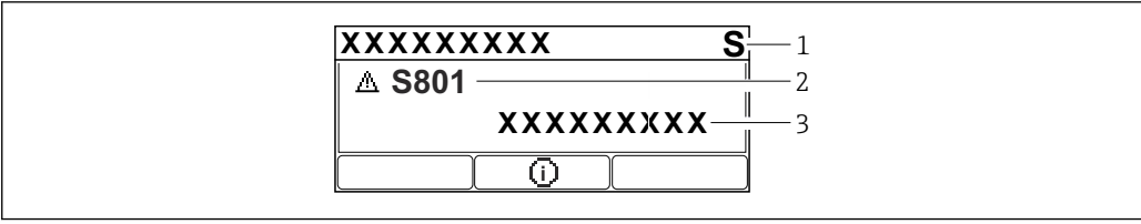
图 16 图形显示屏，带按键 1 状态信号 2 状态图标及诊断事件（开头显示事件类别图标） 3 事件文本
