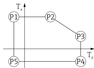
50 316L 外壳，卫生型；过程温度范围：-40 ... +150 °C (-40 ... +302 °F)
