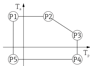
51 316L 外壳，卫生型；过程温度范围：-40 ... +200 °C (-40 ... +392 °F)
