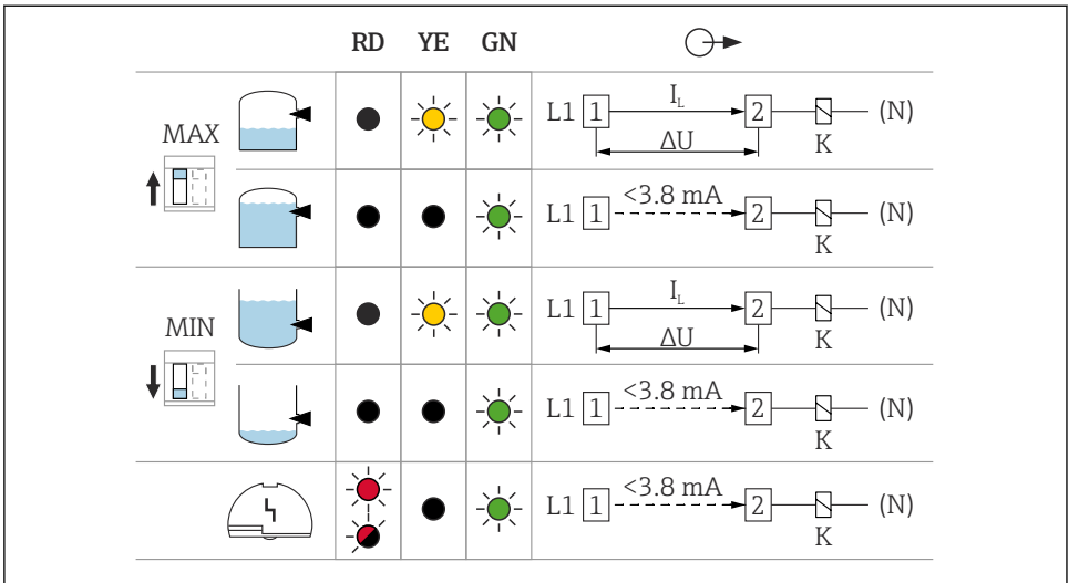
16 Verhalten Schaltausgang und Signalisierung, Elektronikeinsatz FEL61
