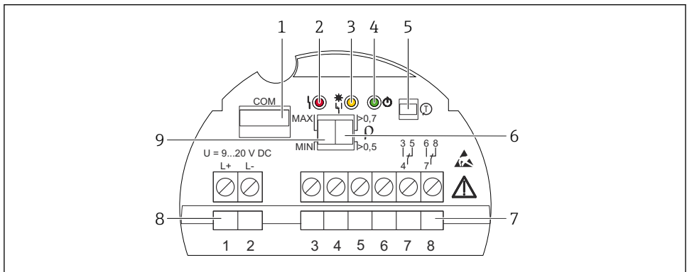
29 Beispiel Elektronikeinsatz FEL64DC
