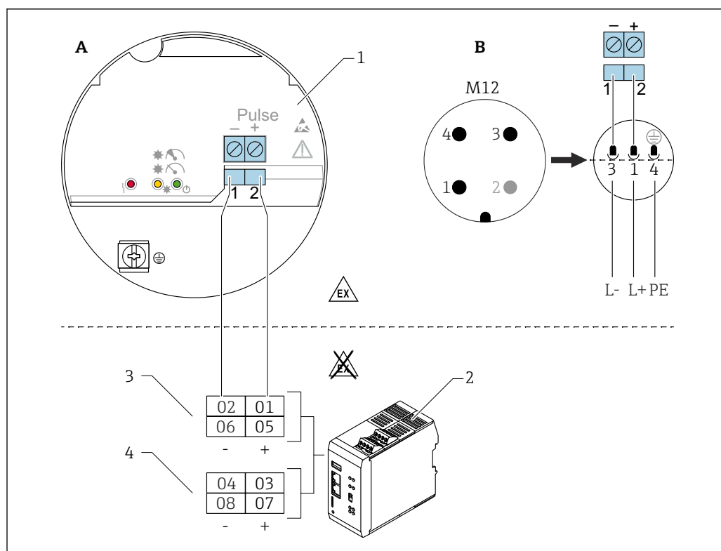
3 Anschlusschema: Anschluss Elektronikmodul FEL60D an den Dichterechner QML51
