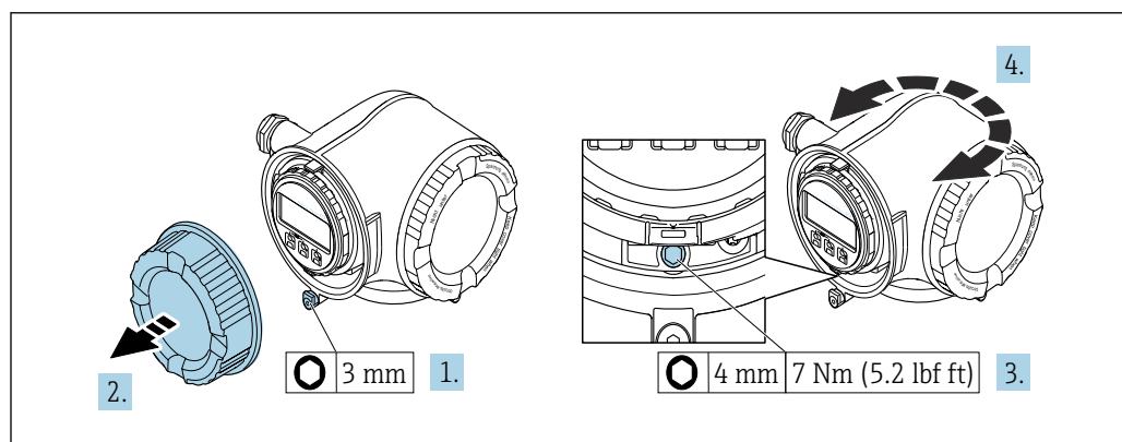
10 Cabezal versión no Ex
