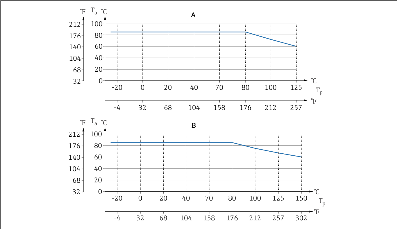
12 I valori valgono per il montaggio verticale senza isolamento. A Tutte le versioni eccetto B B "Versione per alta temperatura" T_p Temperatura di processo T_a Temperatura ambiente
