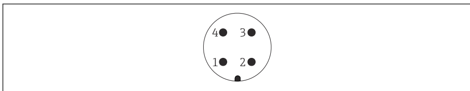
图 14 M12 插头的针脚分配
