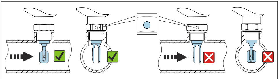
图 12 安装在管道中（注意叉体安装位置和标记）
