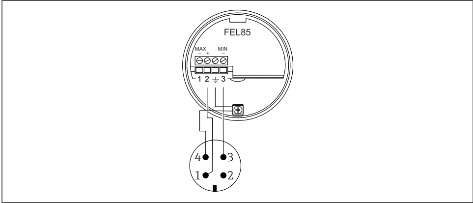
图 16 M12 插头的接线端子分配，低限检测 (MIN) 模式
