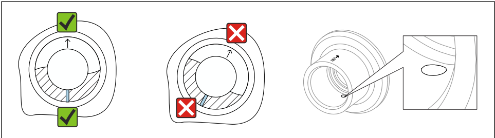
图 10 焊座，带泄漏检测孔
