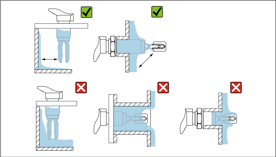
7 安装实例：测量高粘度过程介质
