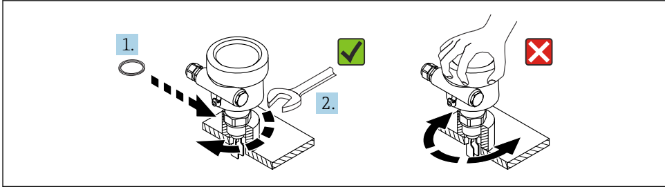
图 13 拧入设备
