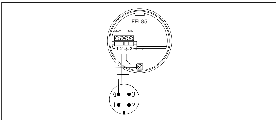
图 15 M12 插头的接线端子分配, 高限检测 (MAX) 模式
