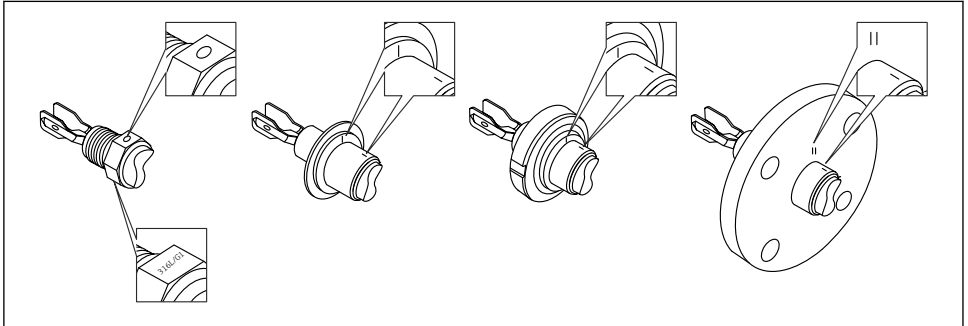
图 11 参照标记水平安装在罐体中时的叉体位置
