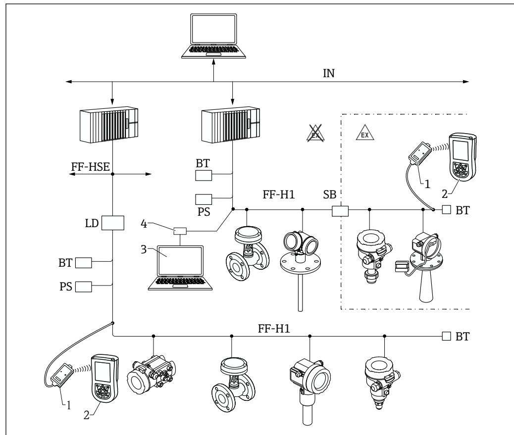
图 42 FOUNDATION Fieldbus 系统架构及其相关部件
