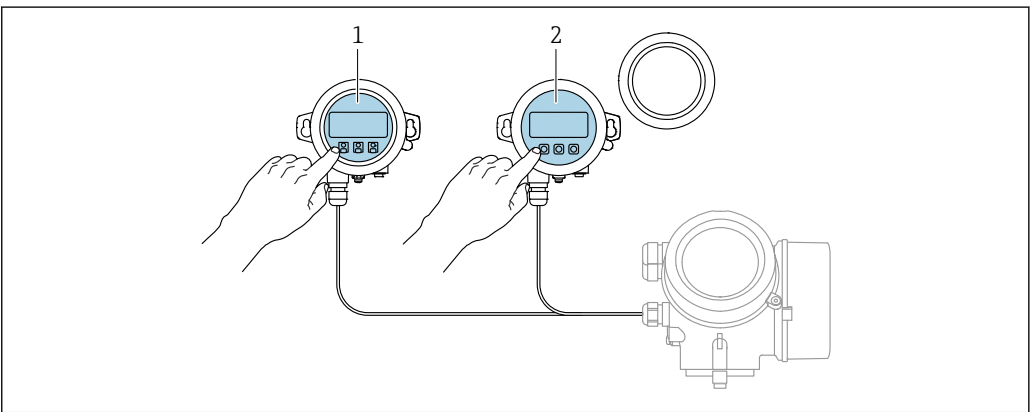
图 37 FHX50 的操作选项
