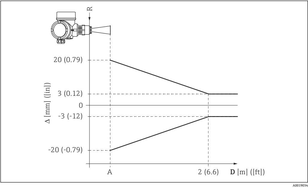
18 近距离测量时的最大测量误差
