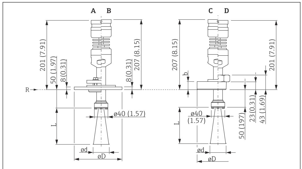
图 35 带喇叭天线的 FMR57 (高温型) 的外形尺寸示意图; 单位: mm (in)
