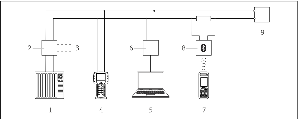
图 40 通过 HART 通信进行远程操作
