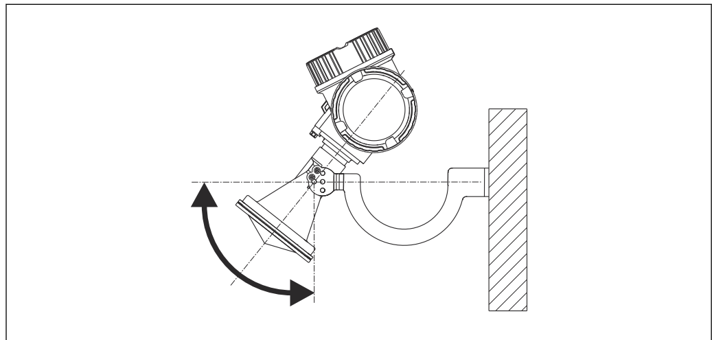
图 21 带安装架的喇叭天线的安装示意图
