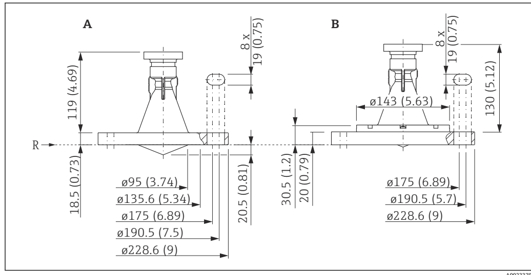
图 32 带 4"/DN100 松套法兰的 FMR56 的外形尺寸示意图。测量单位 mm (in)
