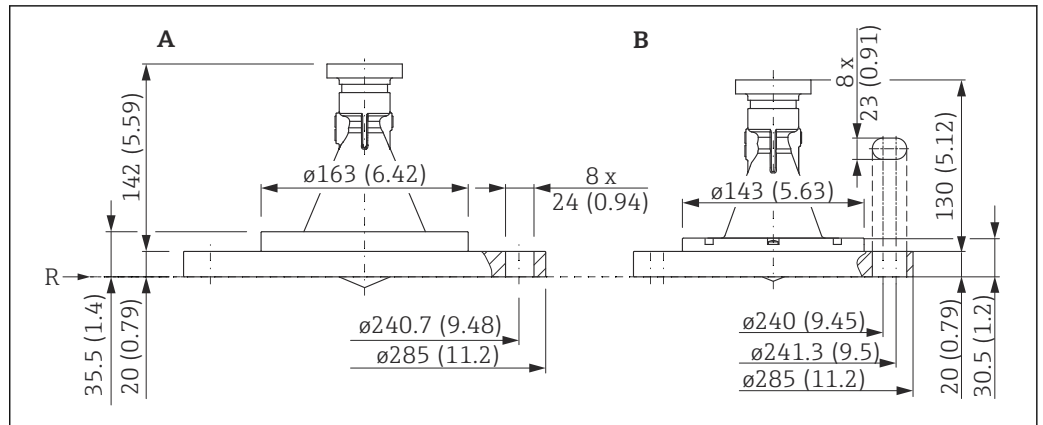
图 33 带 6"/DN150 松套法兰的 FMR56 的外形尺寸示意图。测量单位 mm (in)
