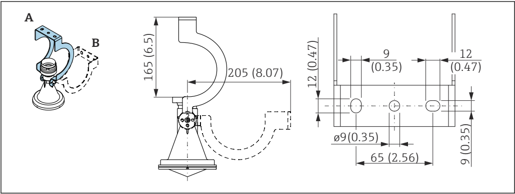
图 30 安装架的外形尺寸示意图。测量单位 mm (in)
