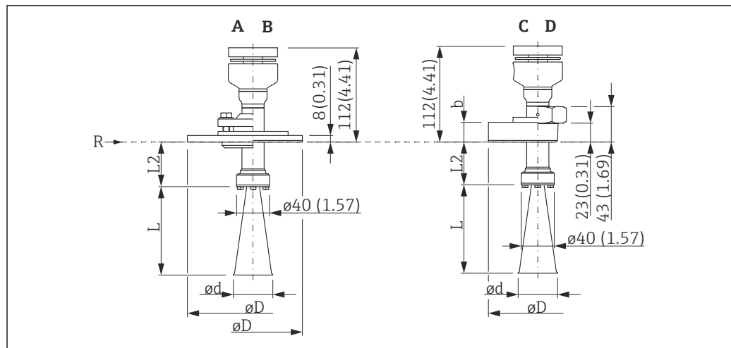
图 34 带喇叭天线的 FMR57 (标准型) 的外形尺寸示意图。测量单位 mm (in)
