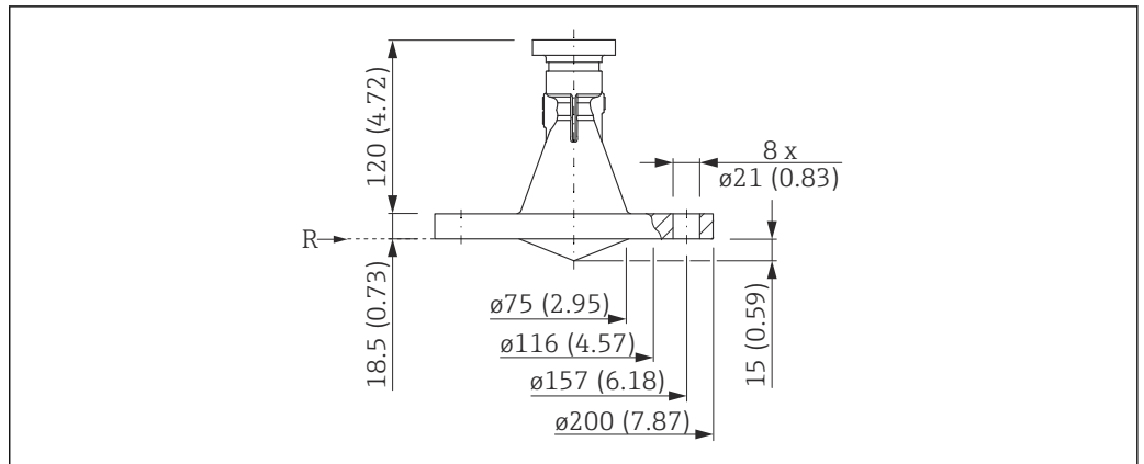
图 31 带 3"/DN80 松套法兰的 FMR56 的外形尺寸示意图。测量单位 mm (in)
