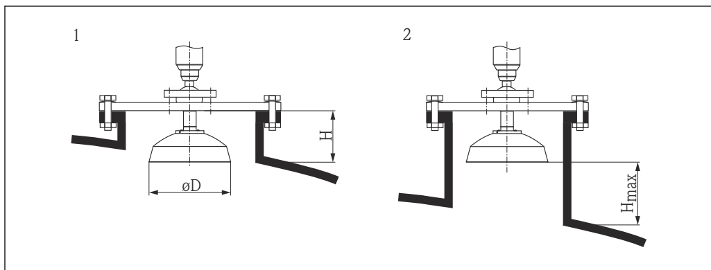
图 23 带抛物面天线的 Micropilot 的安装短管安装示意图
