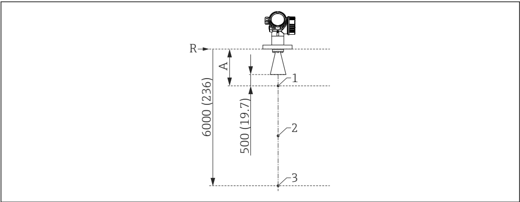
图 46 三点线性标定中的三个标定点的图示说明；单位：mm (in)
