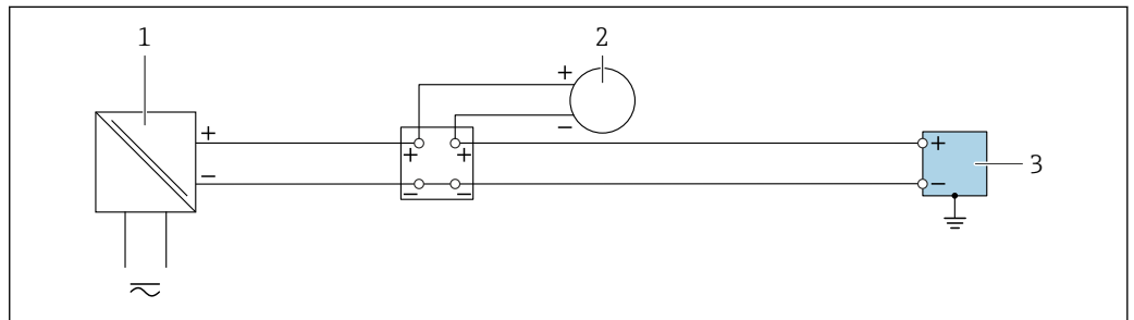
図 23 4～20 mA 電流入力の接続例
