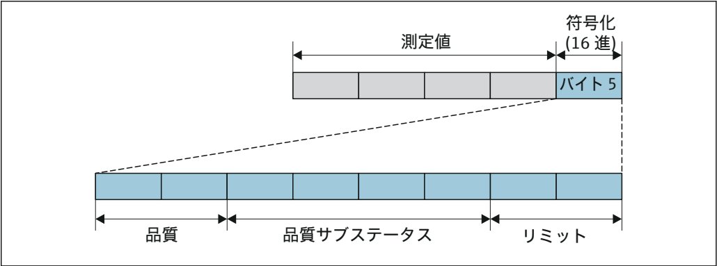
図 41 符号化バイトの構造
