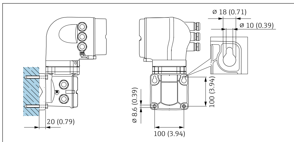
図 15 単位 mm (in)
