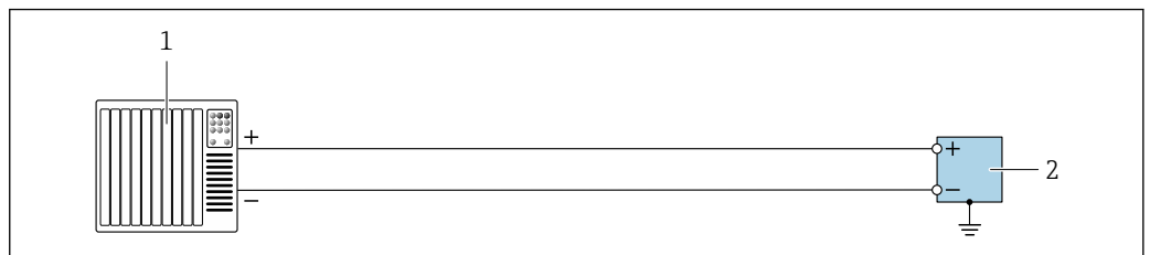
図 24 パルス出力/周波数出力/スイッチ出力（アクティブ）の接続例
