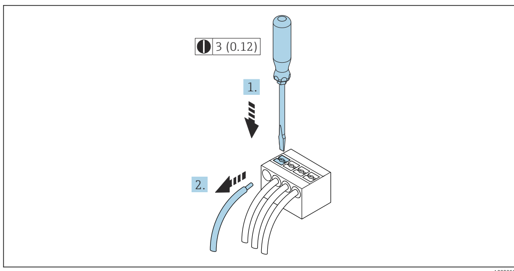
図 20 単位 mm (in)
