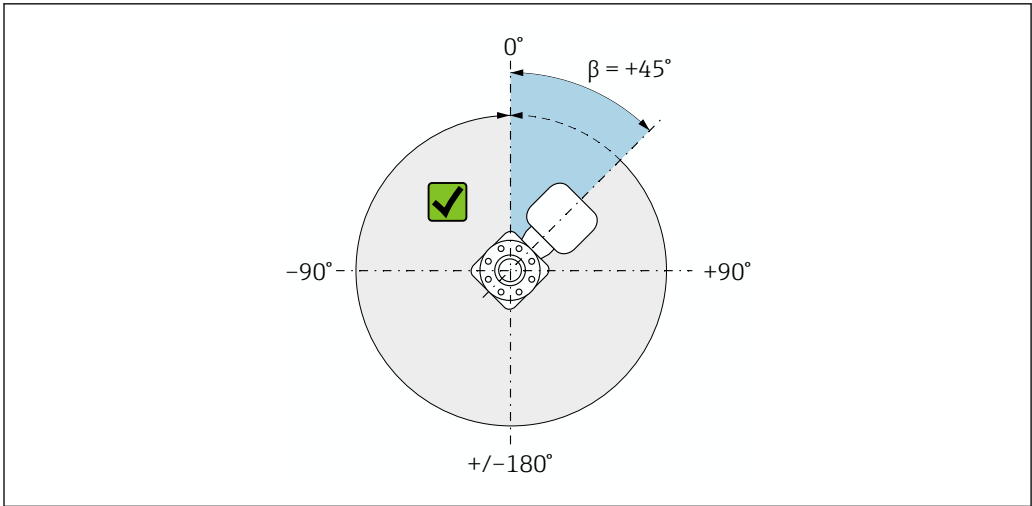
図 10 流れ方向の上面図
