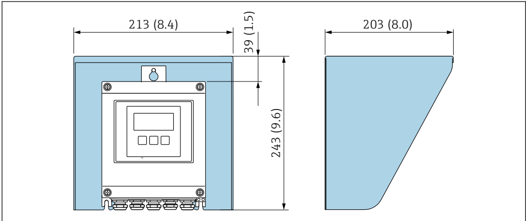
図 11 Proline 500 – デジタル用の日除けカバー、単位 mm (in)
