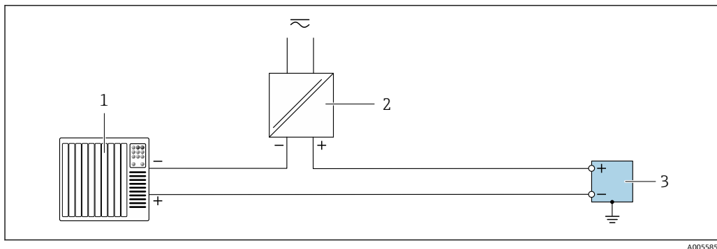
図 25 パルス出力/周波数出力/スイッチ出力（パッシブ）の接続例
