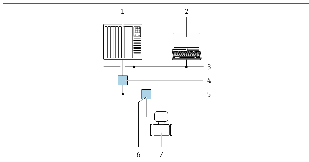
図 33 PROFIBUS PA ネットワークを介したリモート操作のオプション
