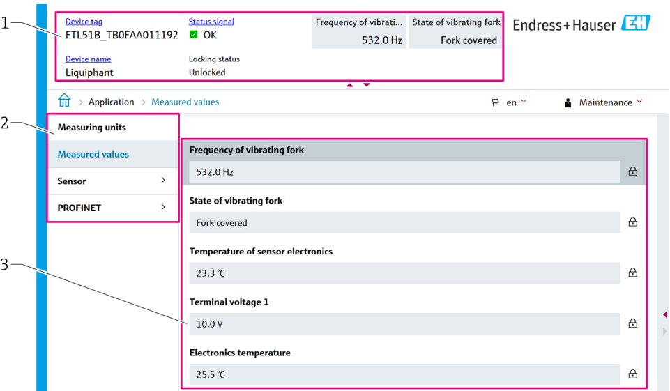
图 25 用户界面示意图
