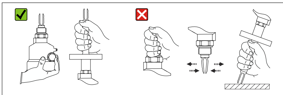
图 1 搬运设备
