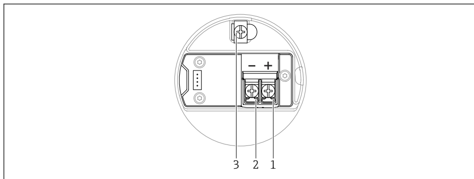
图 17 接线腔内的接线端子和接地端，双腔室外壳（L 型）
