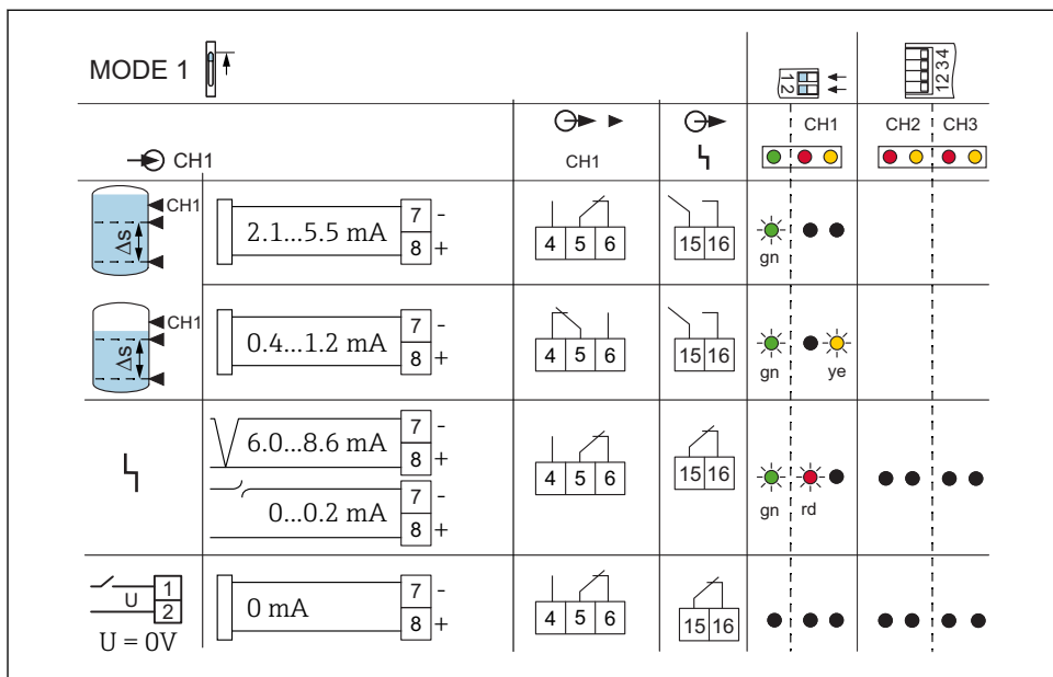
24 Comportament de comutare și semnalizarea erorilor cu curent de eroare H > 2,1 \text{ mA} (FEL56)
