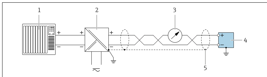
28 Exemple de raccordement pour sortie courant 4 ... 20 mA avec HART (passive)
