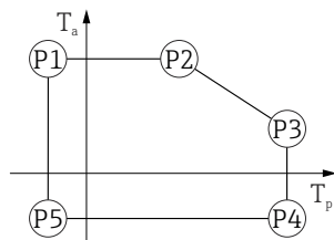
図 25 アルミニウムハウジング ; コーティング ; プロセス温度 -40\sim+200\text{ }^{\circ}\text{C} ( -40\sim+392\text{ }^{\circ}\text{F} )
