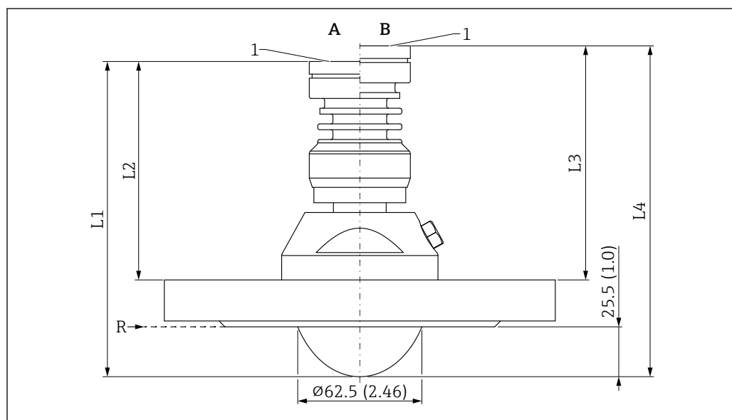
図 52 フラッシュマウントアンテナ (PTFE、80 mm (3 in)、標準フランジおよびエアーパージコネクション付き) の寸法。測定単位 mm (in)
