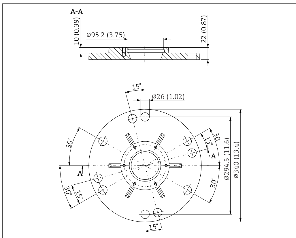
図 46 UNI フランジ 8"/DN200/200A (角度調節器付きアンテナ用) の寸法。測定単位 mm (in)
