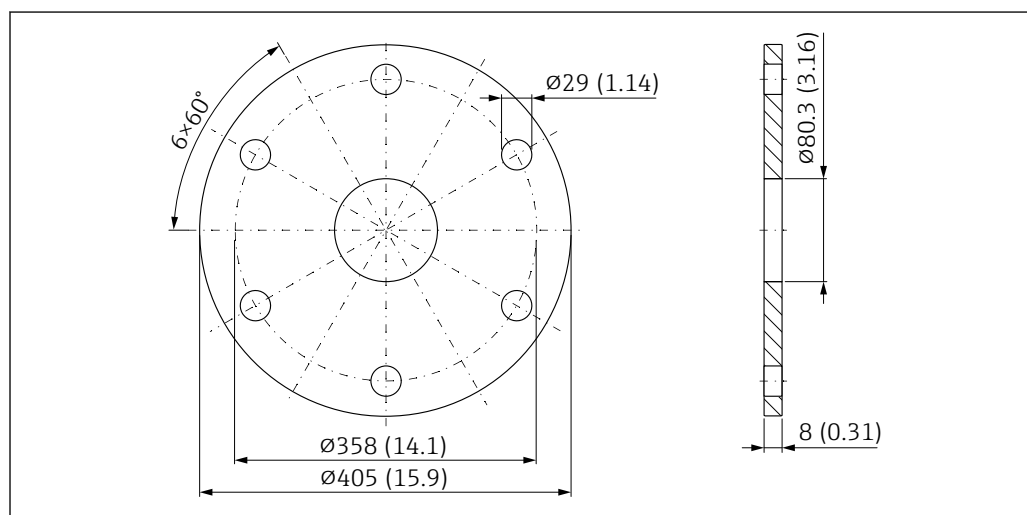
図 55 UNI フランジ 10"/DN250/250A (エアーパージコネクション付き DN80 アンテナ用) の寸法。測定単位 mm (in)
