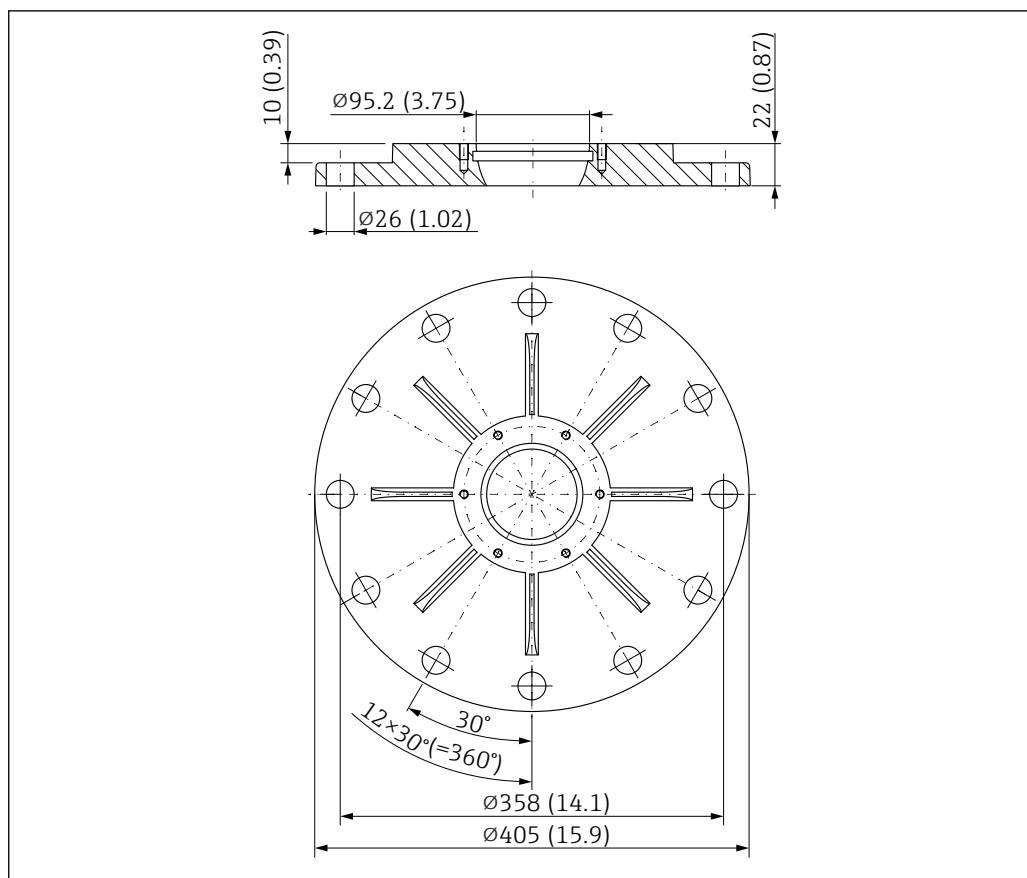
図 60 UNI フランジ 10"/DN250/250A (角度調節器付きアンテナ用) の寸法。測定単位 mm (in)
