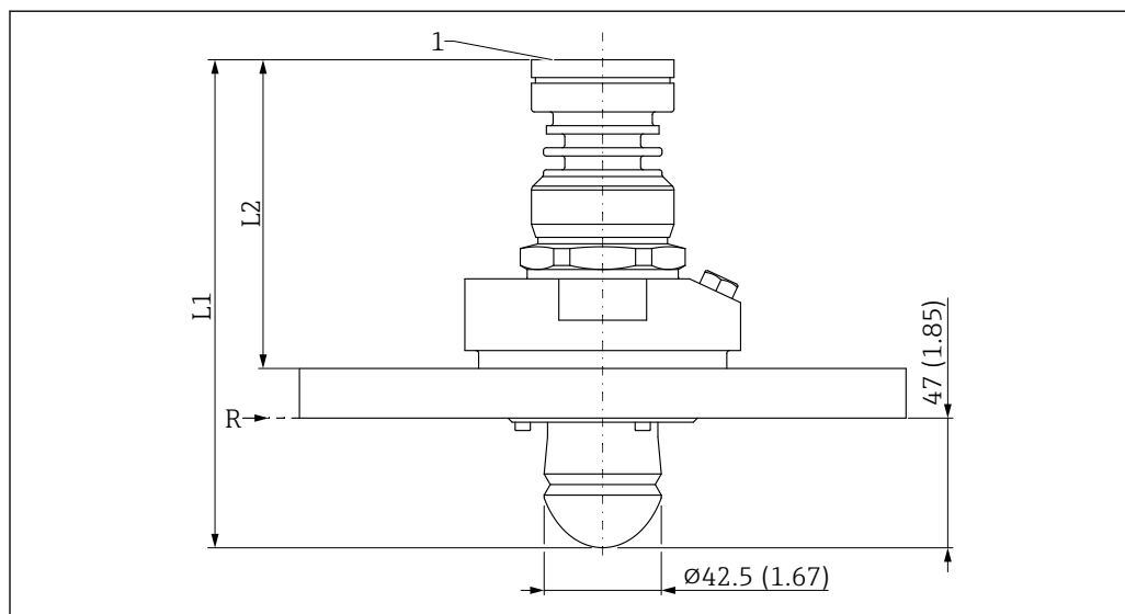
図 48 ドリップオフアンテナ (PTFE、50 mm (2 in)、UNI フランジおよびエアパージコネクション付き) の寸法。測定単位 mm (in)
