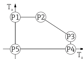
図 22 プラスチックハウジング ; プロセス温度 0～+450 °C (+32～+842 °F)、CSA C/US 認定取得
