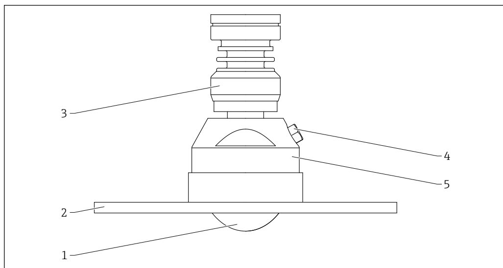
図 65 材質；アンテナ、フラッシュマウント、80 mm (3 in)、UNI フランジおよびパージエア接続付き。測定単位 mm (in)
