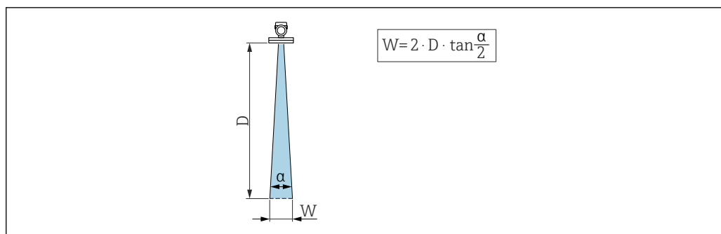
図 12 ビーム放射角 \alpha 、距離 D 、ビーム幅 W の関係
