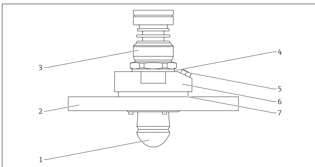
図 63 材質；ドリップオフアンテナ、パージエア接続。測定単位 mm (in)
