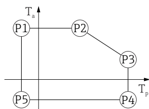
図 19 プラスチックハウジング ; プロセス温度 -40 \sim +280\text{ }^{\circ}\text{C} ( -40 \sim +536\text{ }^{\circ}\text{F} )
