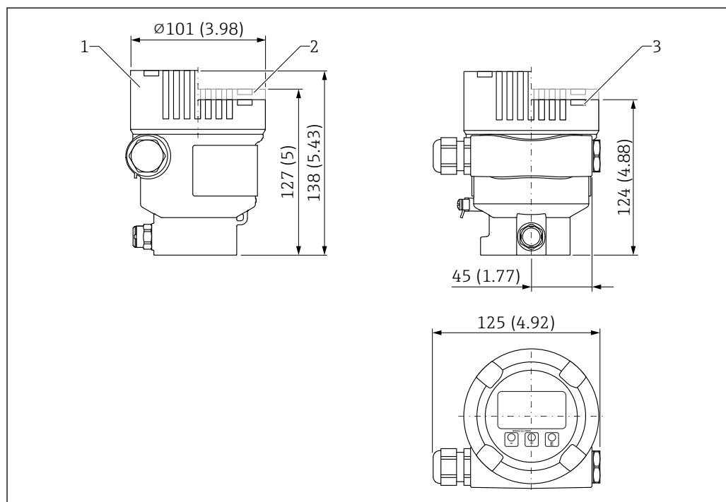
図 37 寸法 ; シングルコンパートメントハウジング (アルミニウム、コーティング) ; M20 カップリングおよびプラグ (プラスチック) 付き。測定単位 mm (in)
