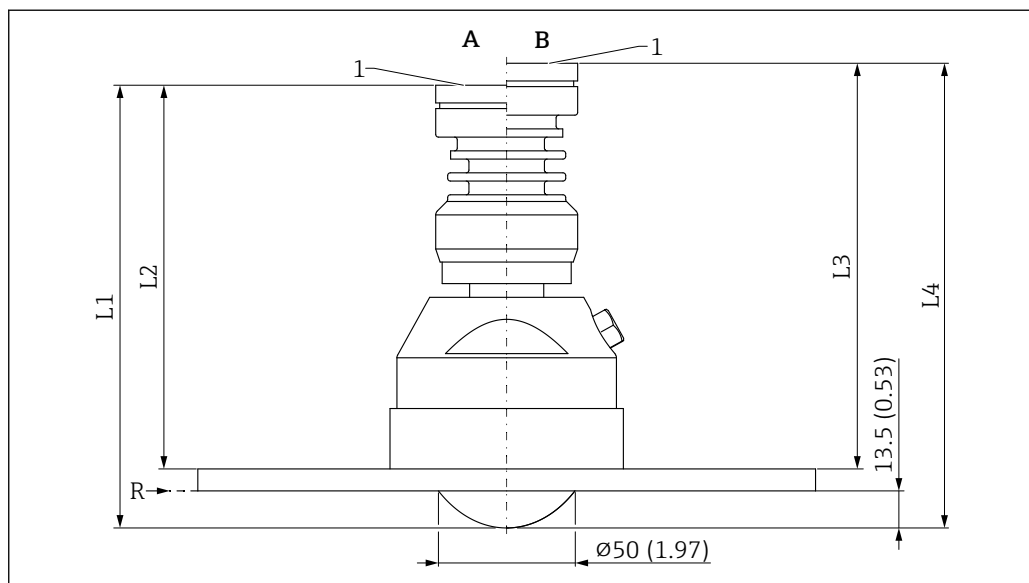
■ 53 フラッシュマウントアンテナ (PTFE、80 mm (3 in)、UNI フランジおよびエアージャコネクション付き) の寸法。測定単位 mm (in)
