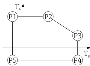
図 34 SUS 316L 相当製ハウジング、サニタリ仕様 ; プロセス温度範囲 : -40 \sim +150^{\circ}\text{C} ( -40 \sim +302^{\circ}\text{F} )
