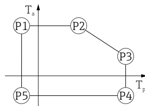
図 28 SUS 316L 相当製ハウジング ; プロセス温度 -40 \sim +80^{\circ}\text{C} ( -40 \sim +176^{\circ}\text{F} )
