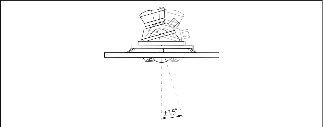
図 10 角度調節器付きフラッシュマウントアンテナ
