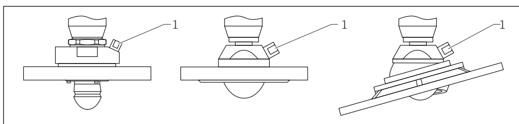
図 11 エアパージアダプタ付きアンテナ
