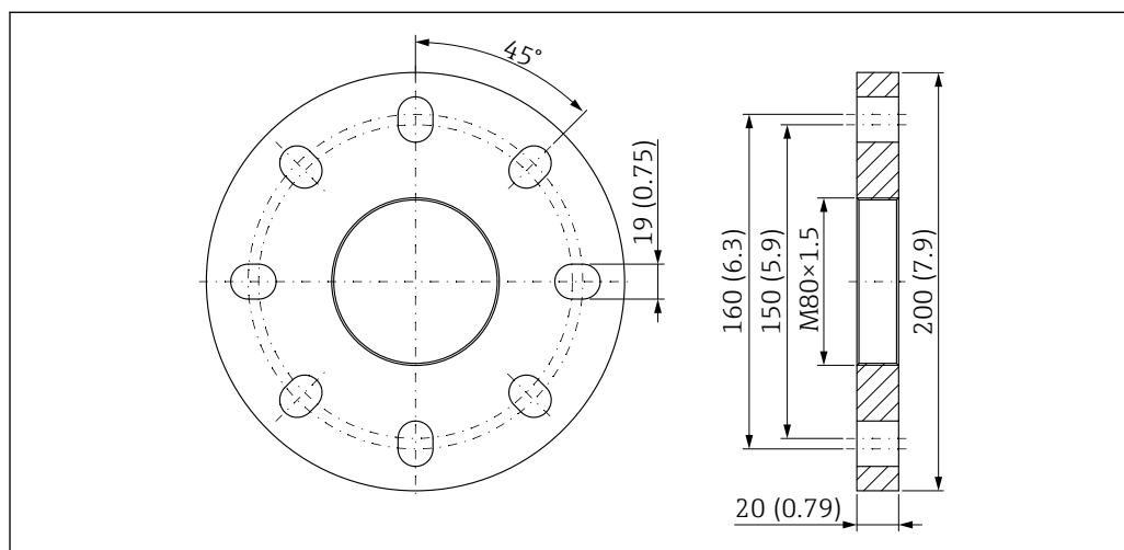
図 49 UNI フランジ 3"/DN80/80A (ドリップオフアンテナ (PTFE、50 mm (2 in)、エアパージコネクション付き) 用)。測定単位 mm (in)
