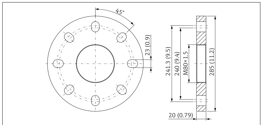
51 UNI フランジ 6"/DN150/150A (ドリップオフアンテナ (PTFE、50 mm (2 in)、エアージェコネクション付き) 用)。測定単位 mm (in)
