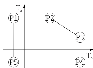
図 35 SUS 316L 相当製ハウジング、サニタリ仕様；プロセス温度 -40\sim+200\text{ }^{\circ}\text{C} ( -40\sim+392\text{ }^{\circ}\text{F} )
