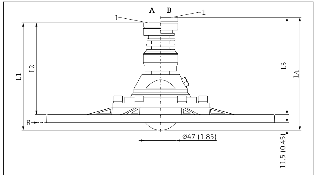
56 フラッシュマウントアンテナ (80 mm (3 in)、UNI フランジ/角度調節器/エアージャコネクション付き) の寸法。測定単位 mm (in)
