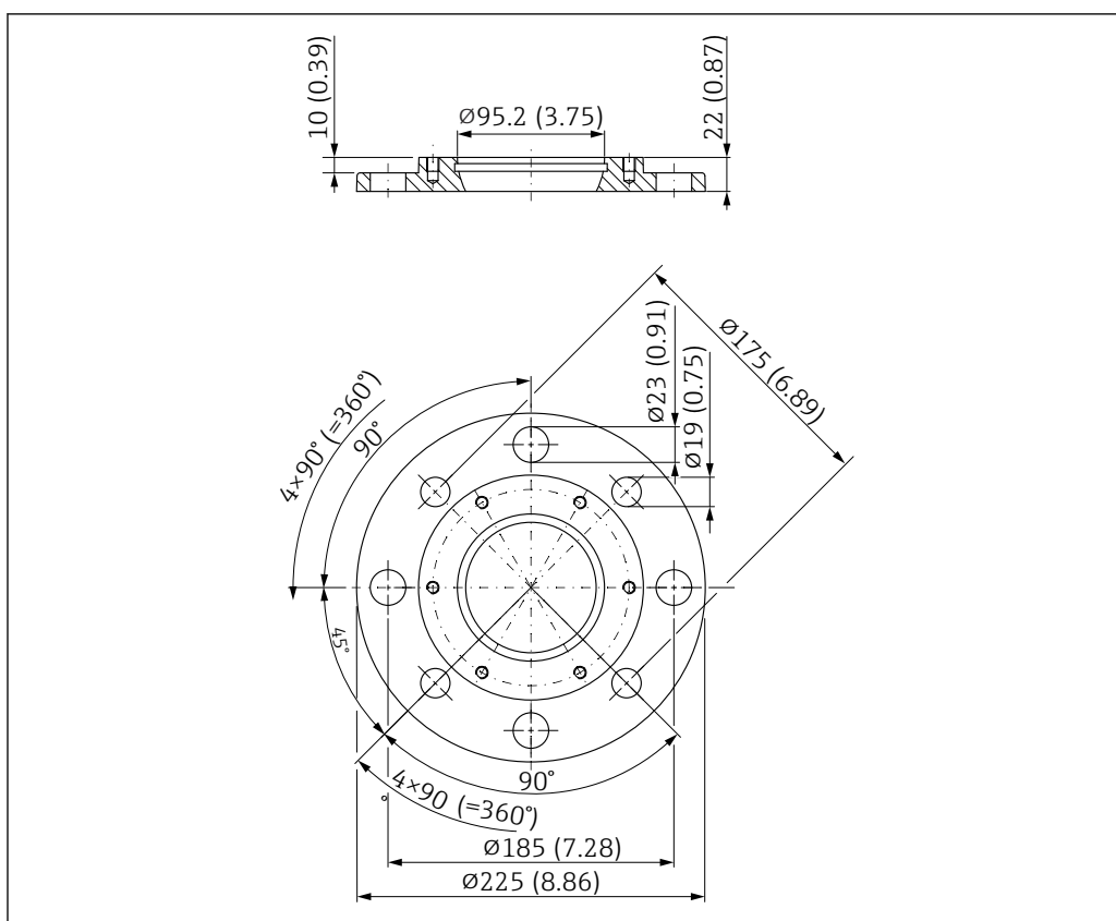
図 44 UNI フランジ UNI 4"/DN100/100A (角度調節器付きアンテナ用) の寸法。測定単位 mm (in)
