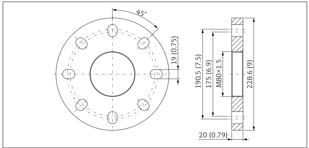
50 UNI フランジ 4"/DN100/100A (ドリップオフアンテナ (PTFE、50 mm (2 in)、エアージェコネクション付き) 用)。測定単位 mm (in)
