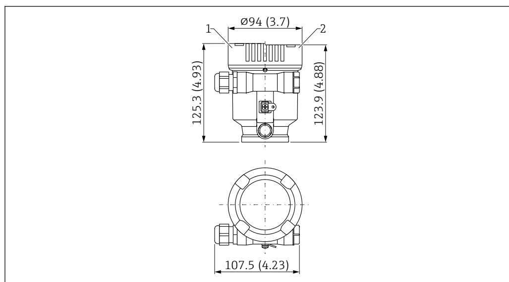
図 36 寸法 ; シングルコンパートメントハウジング (プラスチック) ; M20 カップリングおよびプラグ (プラスチック) 付き。測定単位 mm (in)
