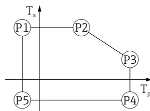
図 21 プラスチックハウジング ; プロセス温度 -40～+450 °C (-40～+842 °F)
