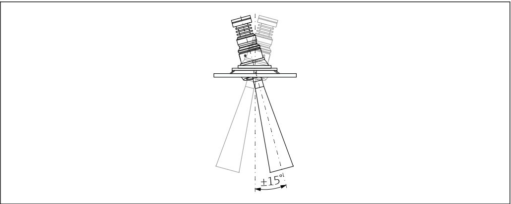
図 9 角度調節器付きホーンアンテナ
