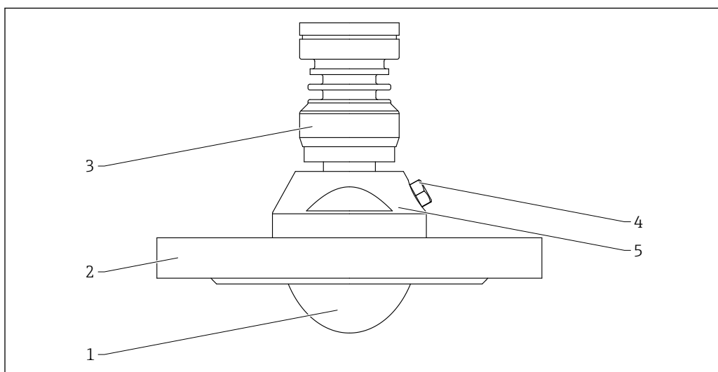
図 64 材質；アンテナ、フラッシュマウント、80 mm (3 in)、フランジおよびパージエア接続付き。測定単位 mm (in)
