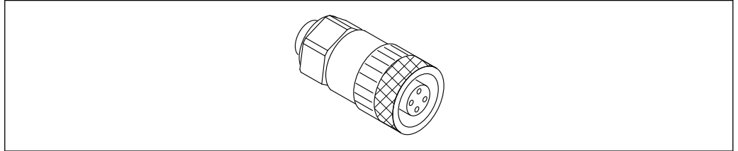
72 M12 ソケット、ケーブル側
