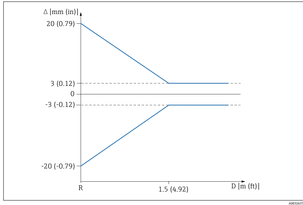
図 8 近範囲アプリケーションにおける最大測定誤差
