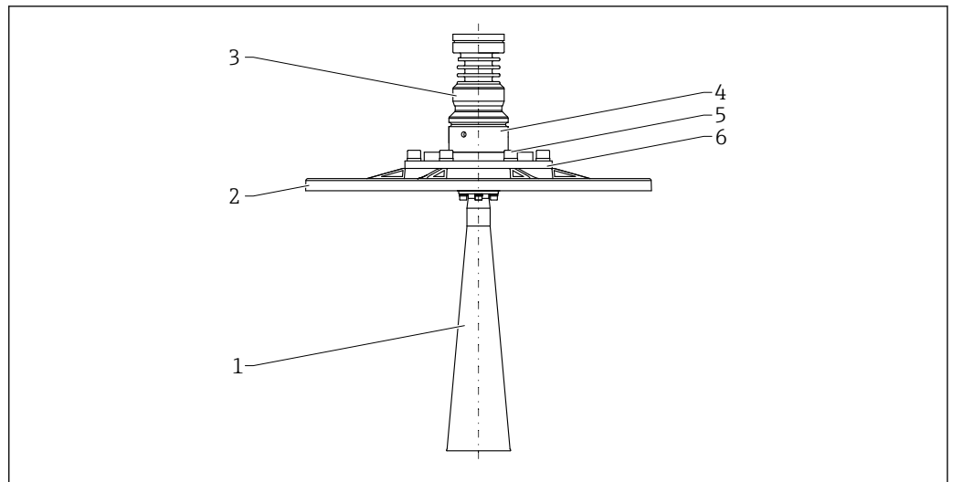
■ 62 材質 ; 65 mm (2.6 in) ホーンアンテナ、UNI フランジおよび角度調節器付き。測定単位 mm (in)
