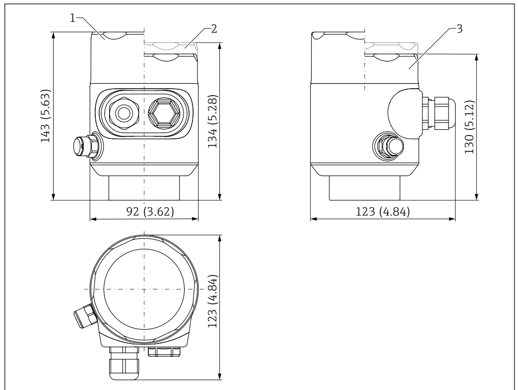
■ 38 寸法；シングルコンパートメントハウジング（SUS 316L 相当、サニタリ仕様）；M20 カップリングおよびプラグ（プラスチック）付き。測定単位 mm (in)
