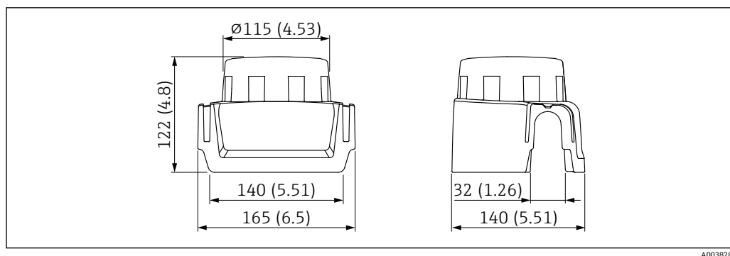
図 71 日除けカバー、プラスチック、XW111 の寸法。測定単位 mm (in)
