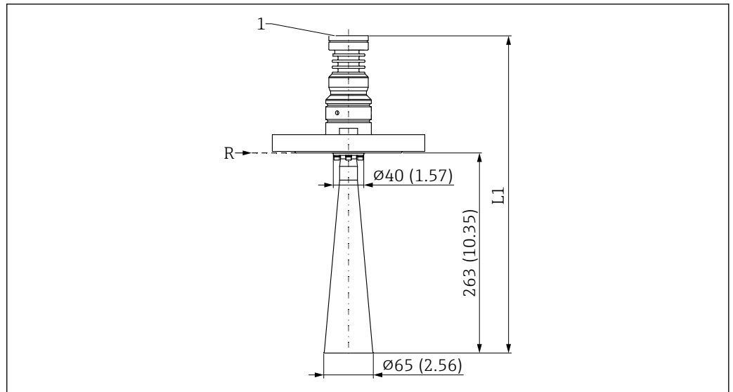
42 DN65 ホーンアンテナ - フランジプロセス接続の寸法。測定単位 mm (in)
