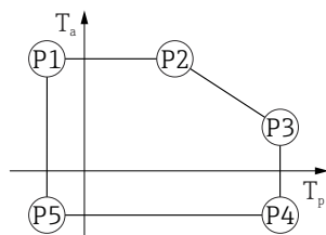
図 23 アルミニウムハウジング ; コーティング ; プロセス温度 -40\sim+80\text{ }^{\circ}\text{C} ( -40\sim+176\text{ }^{\circ}\text{F} )
