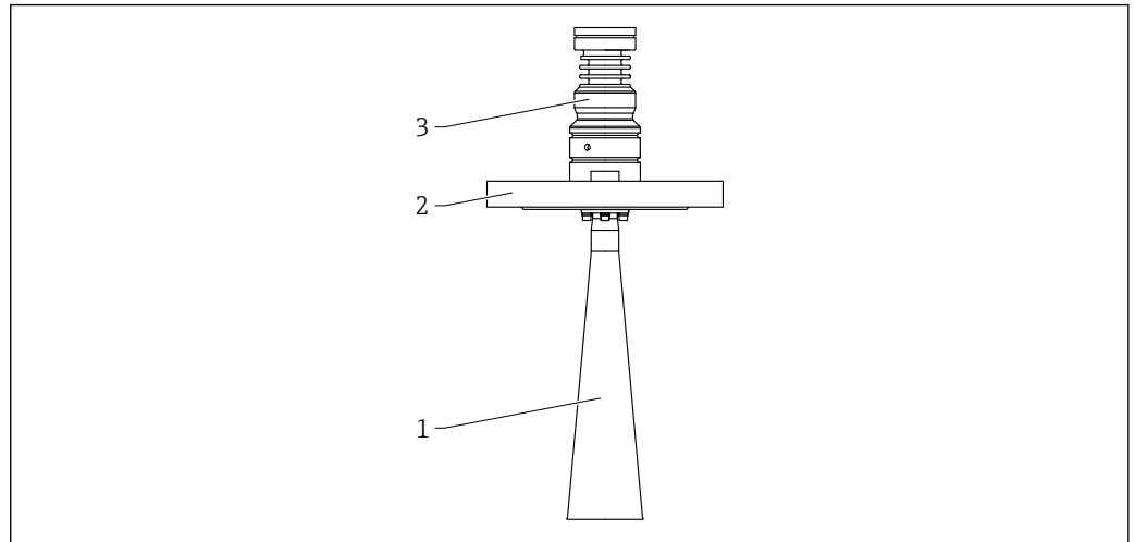
■ 61 材質 ; 65 mm (2.6 in) ホーンアンテナ。測定単位 mm (in)
