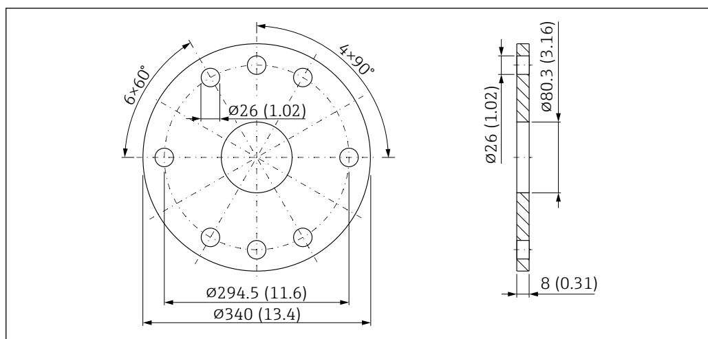
■ 54 UNI フランジ 8"/DN200/200A (エアージャコネクション付き DN80 アンテナ用) の寸法。測定単位 mm (in)
