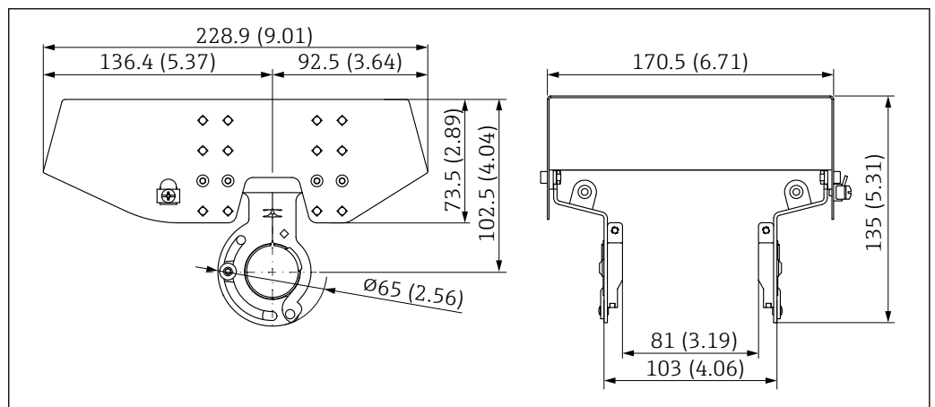
図 70 日除けカバー、SUS 316L 相当、XW112 の寸法。測定単位 mm (in)
