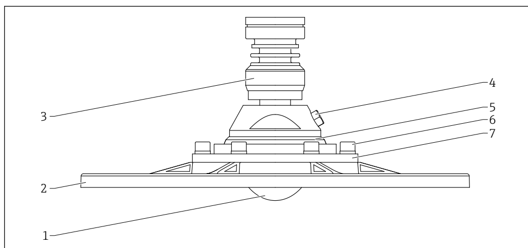
図 66 材質；アンテナ、フラッシュマウント、80 mm (3 in)、UNI フランジ/角度調節器/パージエア接続付き
