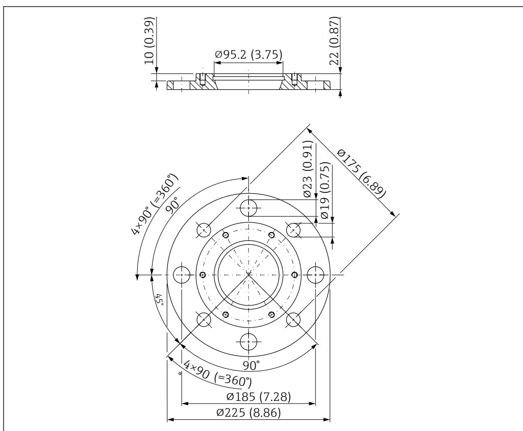
図 57 UNI フランジ UNI 4"/DN100/100A (角度調節器付きアンテナ用) の寸法。測定単位 mm (in)
