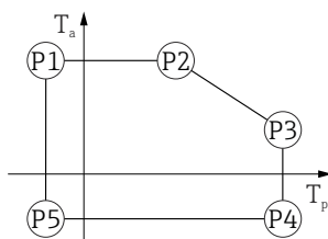
図 33 SUS 316L 相当製ハウジング、サニタリ仕様 ; プロセス温度 -40 \sim +80^{\circ}\text{C} ( -40 \sim +176^{\circ}\text{F} )
