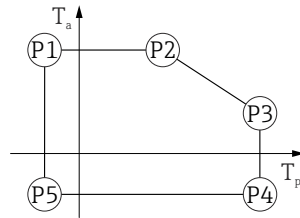
図 15 プラスチックハウジング ; プロセス温度 -40～+150 °C (-40～+302 °F)
