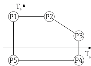
図 13 プラスチックハウジング ; プロセス温度 -40～+80 °C (-40～+176 °F)
