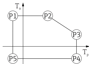
図 24 アルミニウムハウジング ; コーティング ; プロセス温度 -40\sim+150\text{ }^{\circ}\text{C} ( -40\sim+302\text{ }^{\circ}\text{F} )
