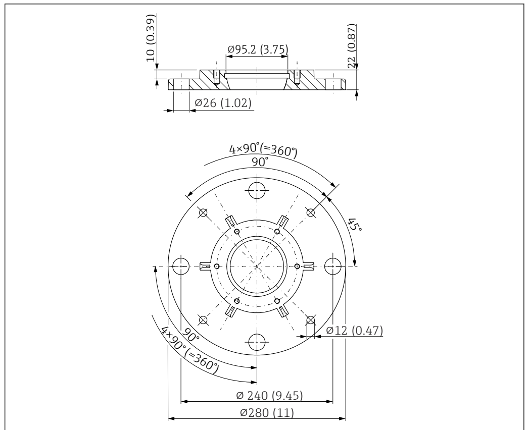
図 58 UNI フランジ 6"/DN150/150A (角度調節器付きアンテナ用) の寸法。測定単位 mm (in)
