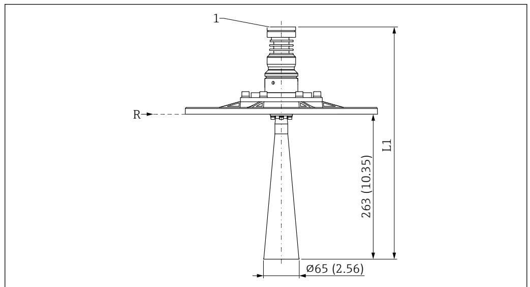
43 DN65 ホーンアンテナ（UNI フランジおよび角度調節器付き）の寸法。測定単位 mm (in)
