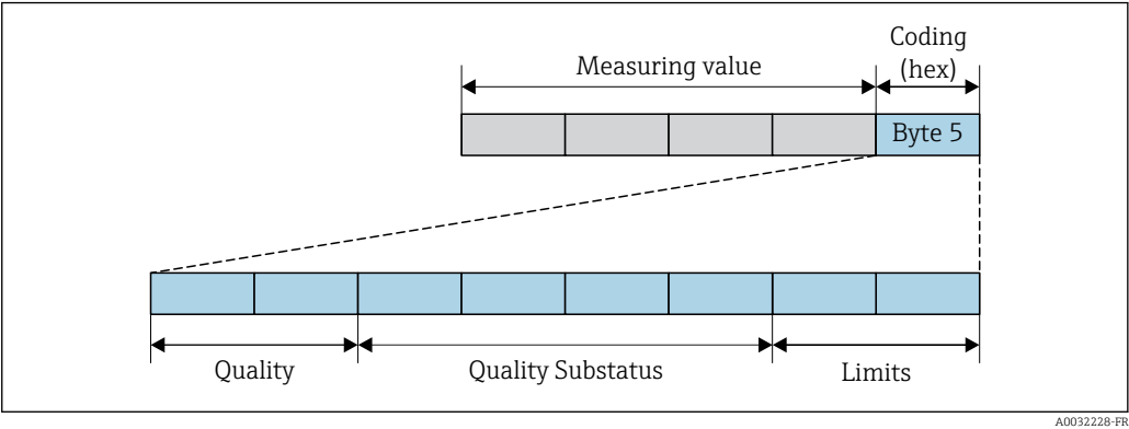
39 Structure de l'octet de codage
