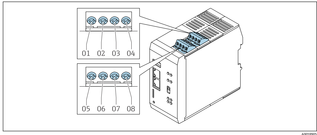
図 34 パルスおよびアナログ入力
