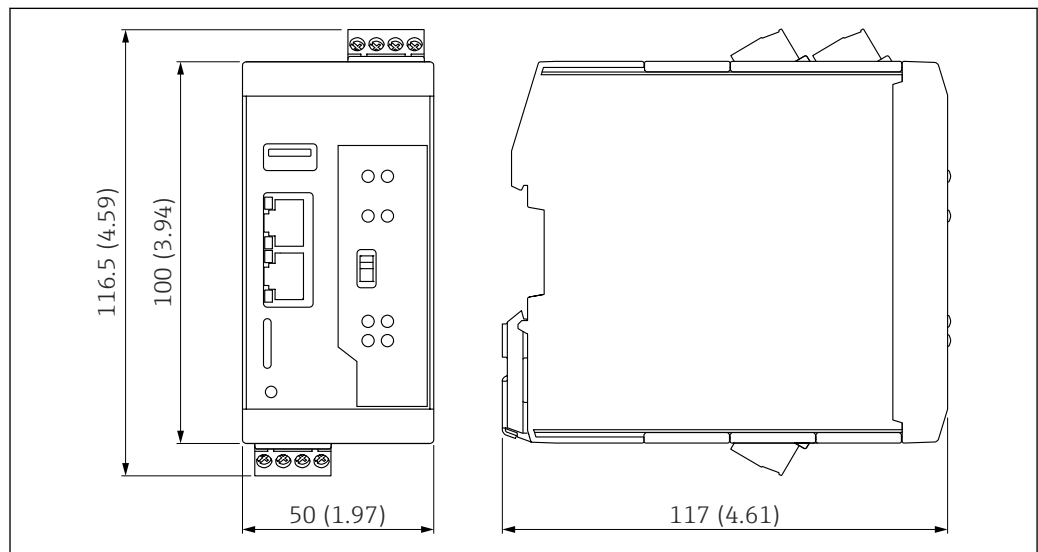
図 35 寸法。測定単位 mm (in)
