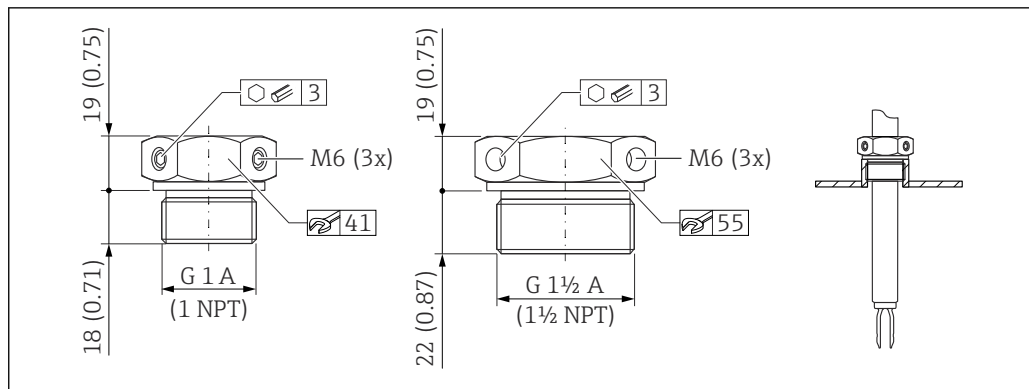
図 42 スライディングスリーブ (大気圧用 : p_e = 0 MPa (0 psi))。測定単位 mm (in)
