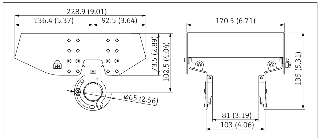
40 日除けカバー、SUS 316L 相当、XW112 の寸法。測定単位 mm (in)
