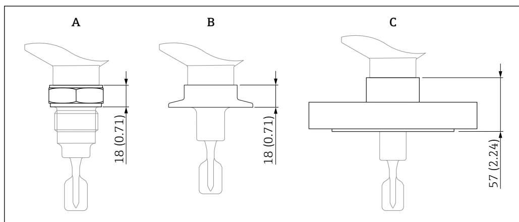
図 22 プロセス接続の最大高さ仕様。測定単位 mm (in)
