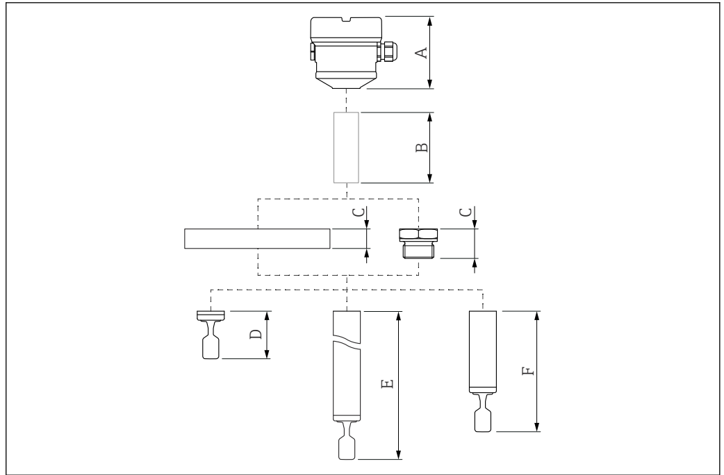
図 13 本体高さを計算するための構成部品
