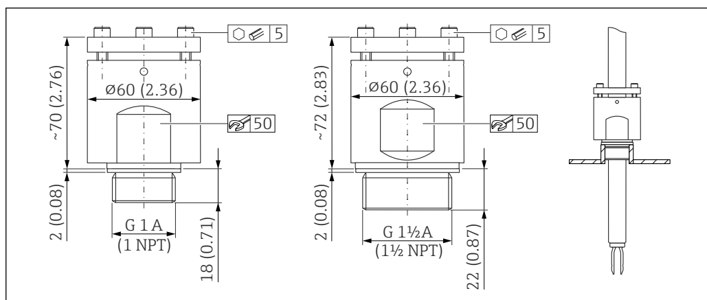
図 43 高圧用スライディングスリーブ。測定単位 mm (in)
