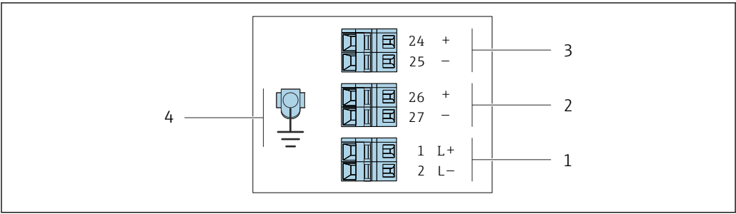
6 Affectation des bornes 4-20 mA HART avec sortie impulsion/fréquence/tor
