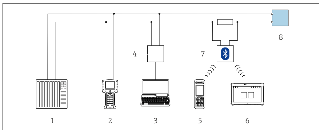
16 Options pour la configuration à distance via protocole HART
