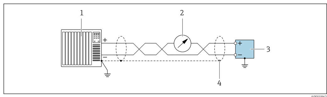
10 Exemple de raccordement pour sortie courant 4 ... 20 mA avec HART (active)
