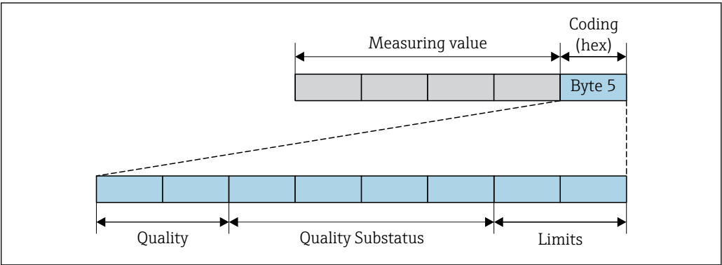
41 Структура байта состояния
