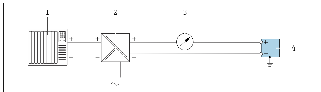
22 Пример подключения для токового выхода 4 до 20 мА (пассивного)
