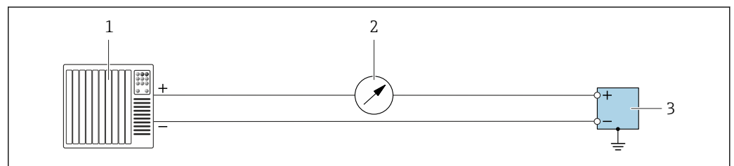
21 Пример подключения для токового выхода 4 до 20 мА (активного)
