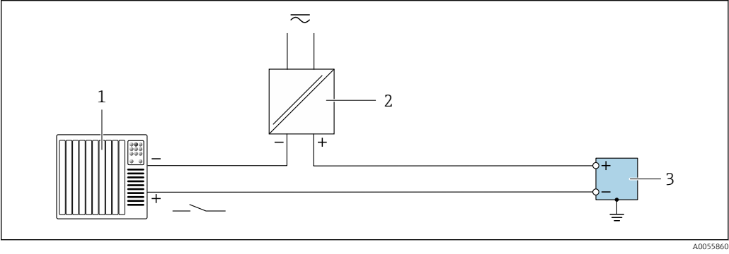
27 Пример подключения для входного сигнала состояния
