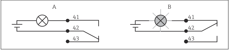
12 Tavsiye edilen arıza emniyetli alarm bağlantı anahtarı
