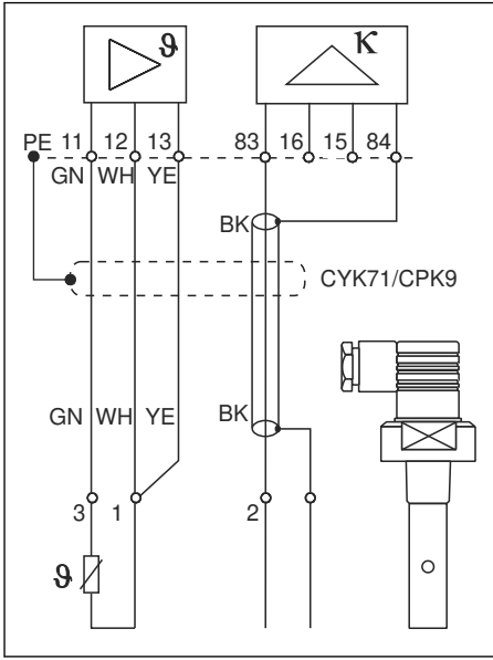
10 İletken sensörlerin bağlantısı
