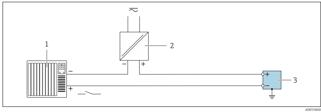
24 Esempio di collegamento per ingresso di stato
