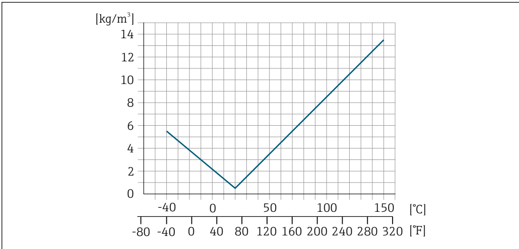
41 Regolazione della densità in campo, ad es. a +20 \text{ }^\circ\text{C} ( +68 \text{ }^\circ\text{F} )
