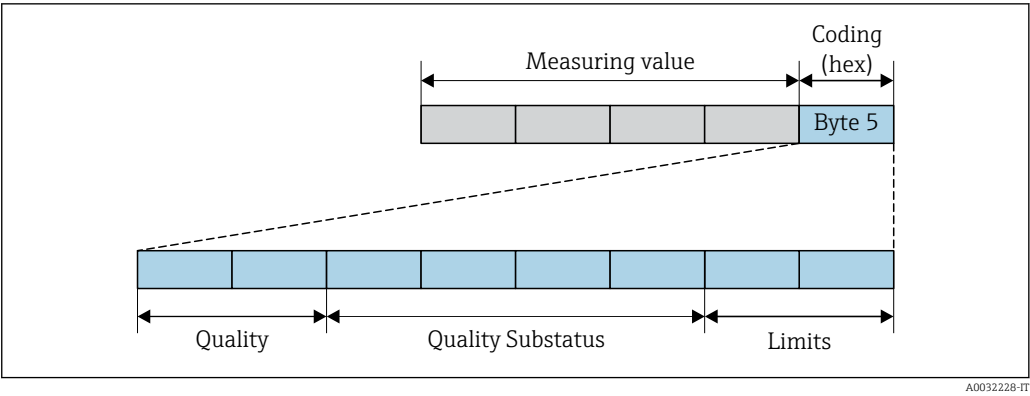
38 Struttura del byte di codifica
