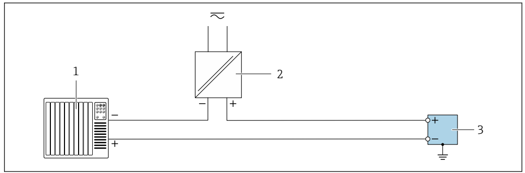
图 2 接线实例：脉冲输出/频率输出/开关量输出（无源）
