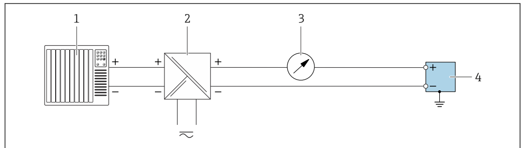
图 1 接线实例：4 ... 20 mA 电流输出（无源）
