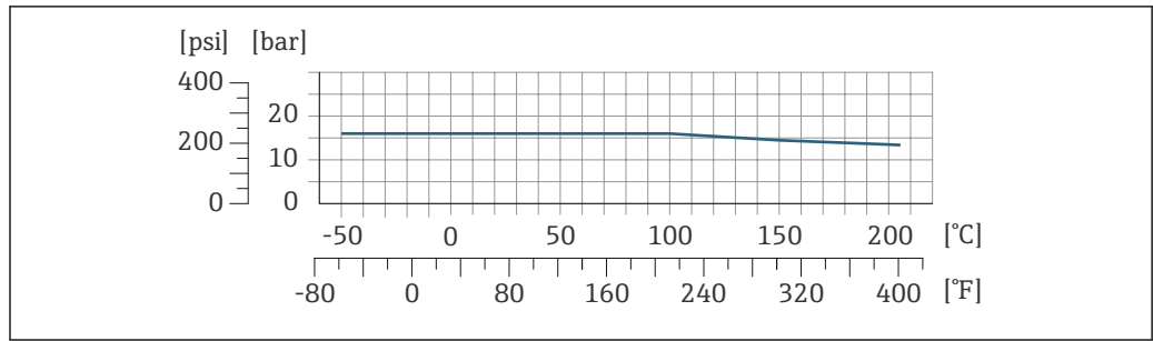
图 17 连接部件材质: 1.4404 (316/316L)
