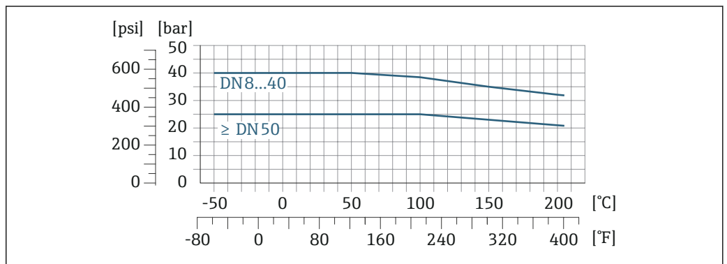
图 16 连接部件材质: 1.4404 (316/316L)
