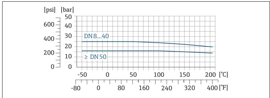
图 11 连接部件材质: 1.4404 (316/316L)
