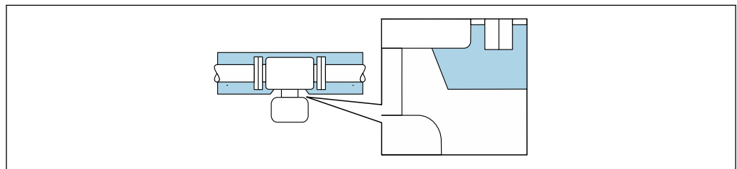
图 19 延长颈上无保温层覆盖
