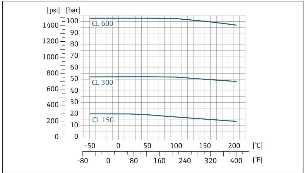
图 9 法兰材质: Alloy C22 合金
