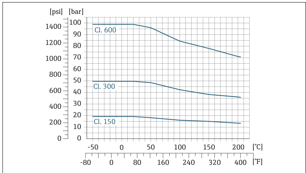
图 8 法兰材质: 1.4404 (F316/F316L)
