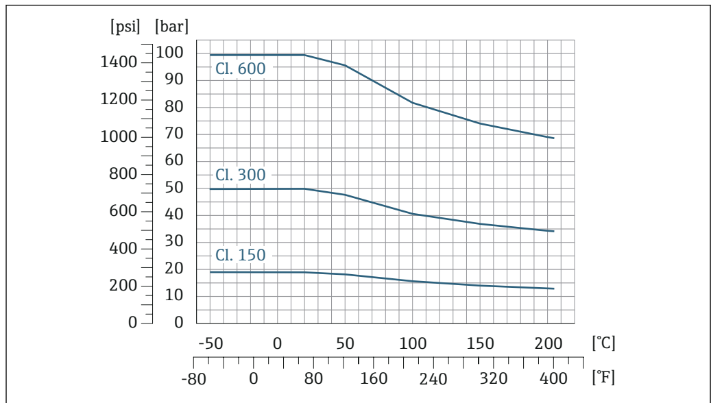
图 13 法兰材质: 1.4301 (F304) ; 接液部件材质: Alloy C22 合金
