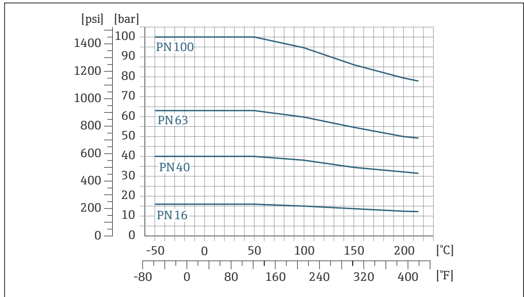
图 7 法兰材质: 1.4404 (F316/F316L) 、 Alloy C22 合金
