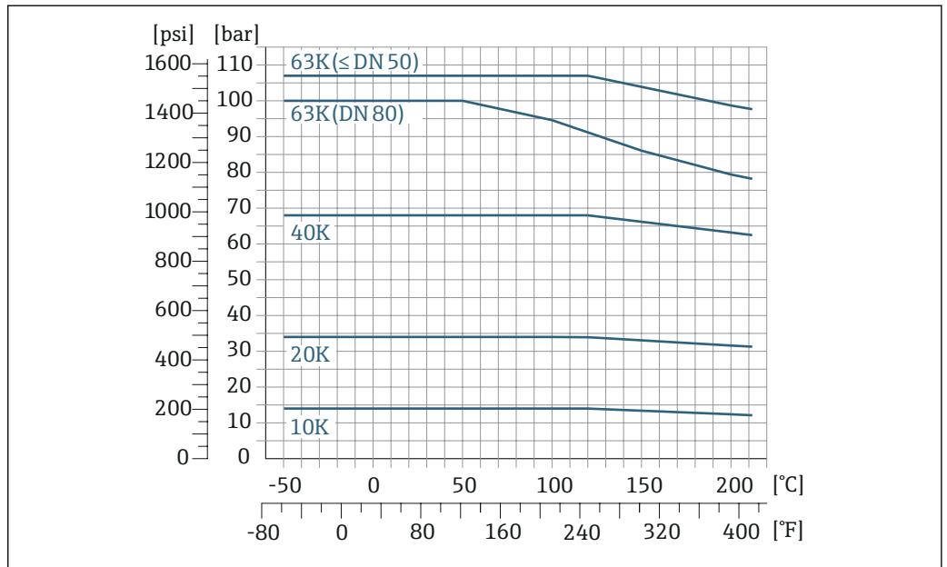
图 10 法兰材质: 1.4404 (F316/F316L)、Alloy C22 合金
