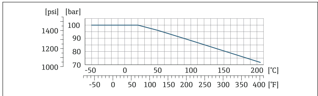
图 18 连接部件材质: 1.4404 (316/316L)
