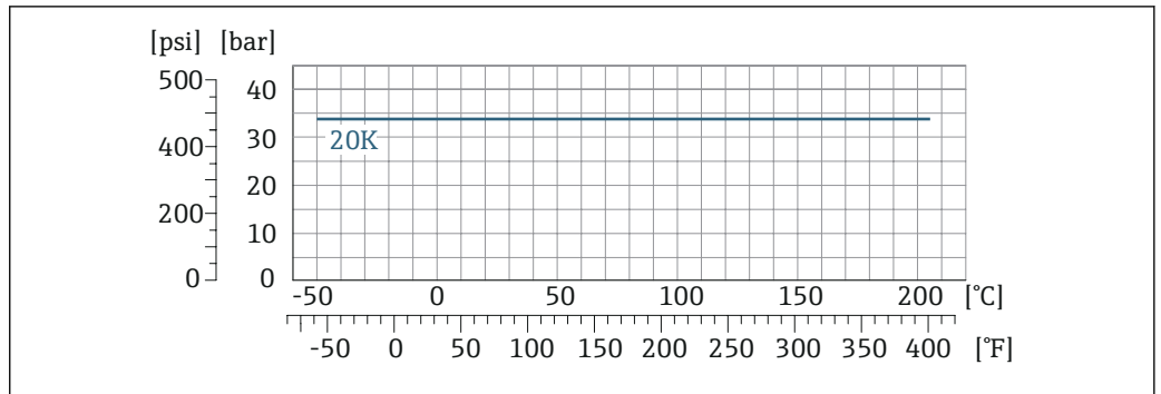
图 14 法兰材质: 1.4301 (F304) ; 接液部件材质: Alloy C22 合金
