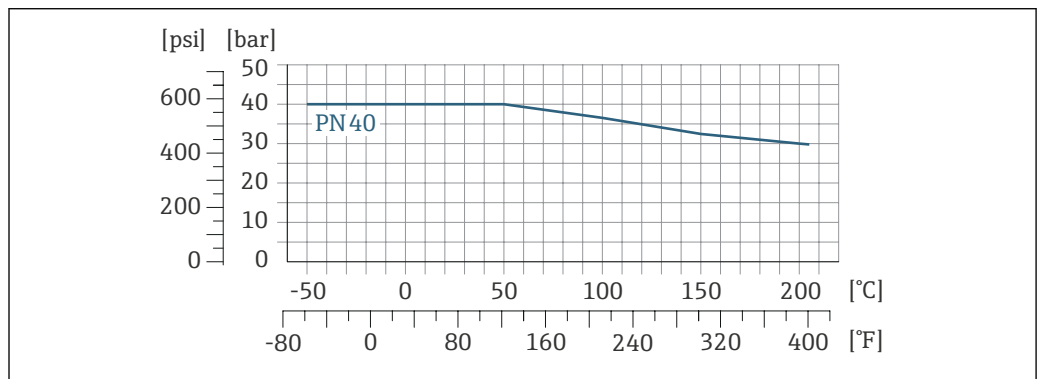
图 12 法兰材质: 1.4301 (F304) ; 接液部件材质: Alloy C22 合金
