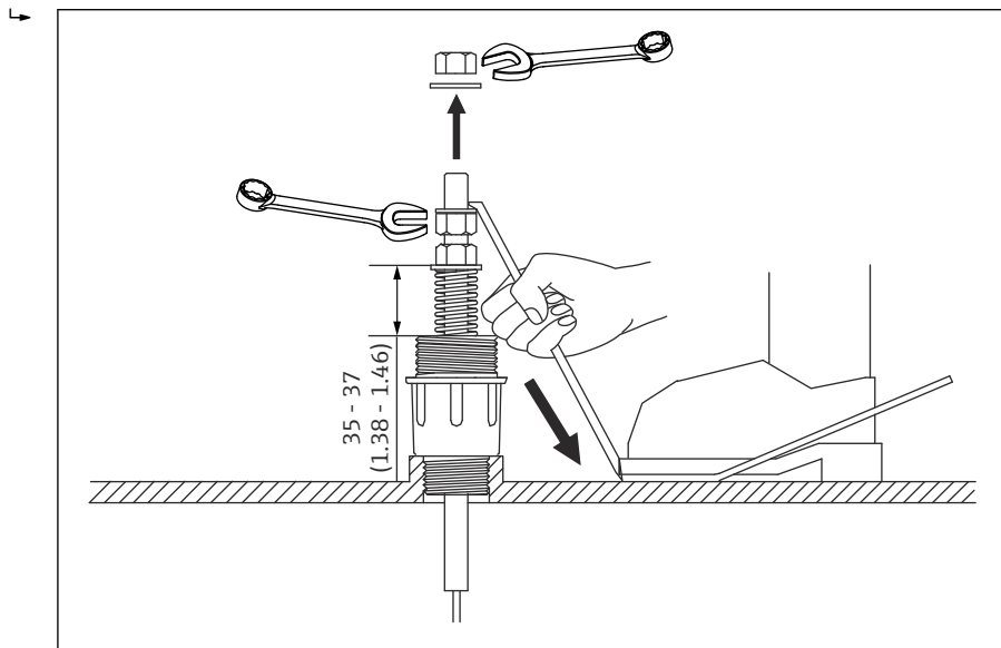
26 Installation med topanker 2. Måleenhed mm (in)
