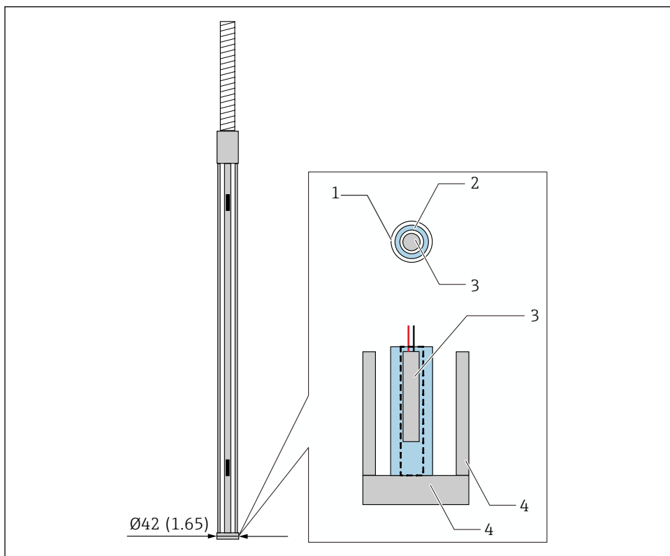
12 Bundfølerens design. Måleenhed mm (in)
