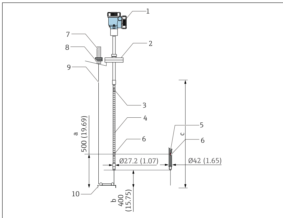
24 Topankermetoden. Måleenhed mm (in)
