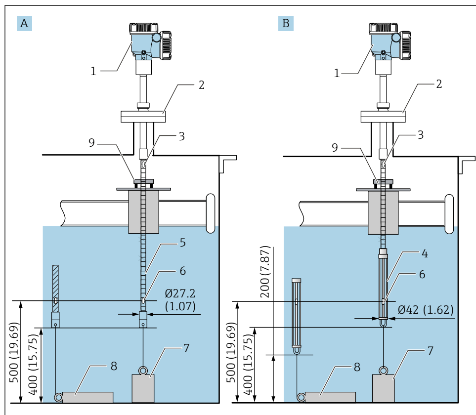
31 Styrerings- og forankringsvægtmetoden. Måleenhed mm (in)
