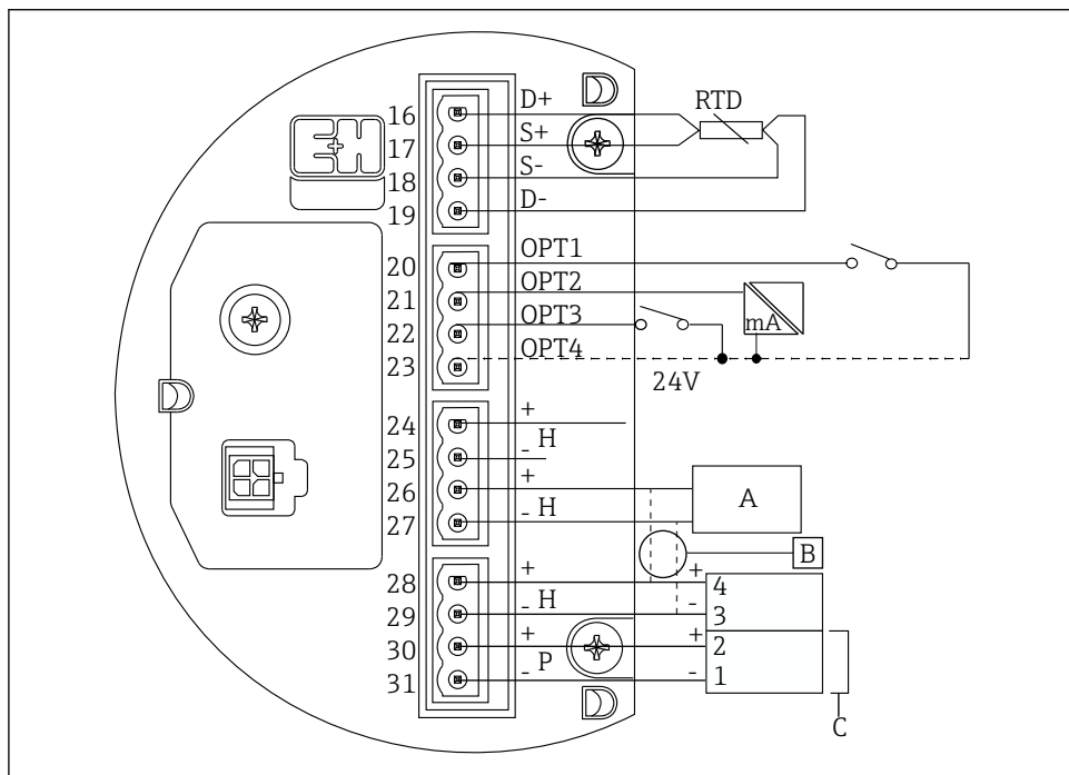
38 (Egensikre) klemmer på NRF590
