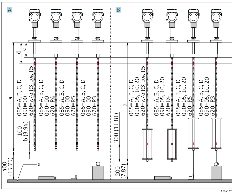
10 Placing for element nr. 1 på NMT81 baseret på installationsmetoden
