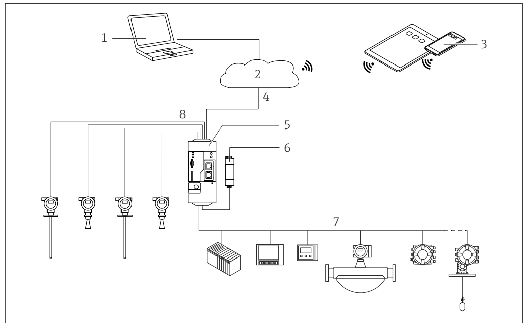
图 7 Fieldgate FXA42 的系统架构 (Modbus RS485 通信)
