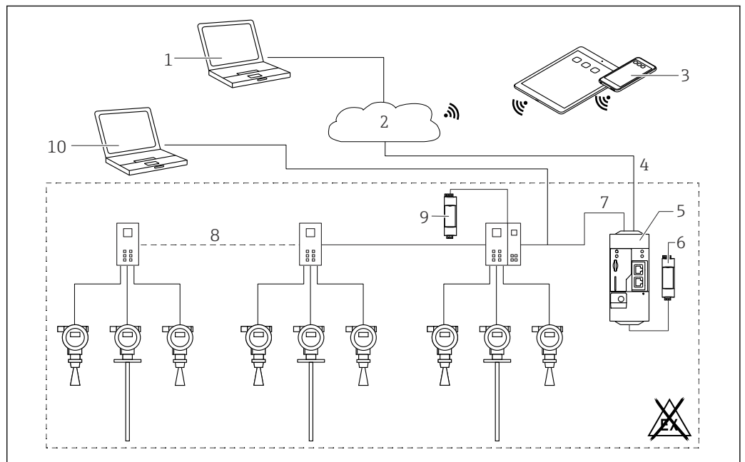
图 6 Fieldgate FXA42 的系统架构 (带 HART 点对点多路复用器)
