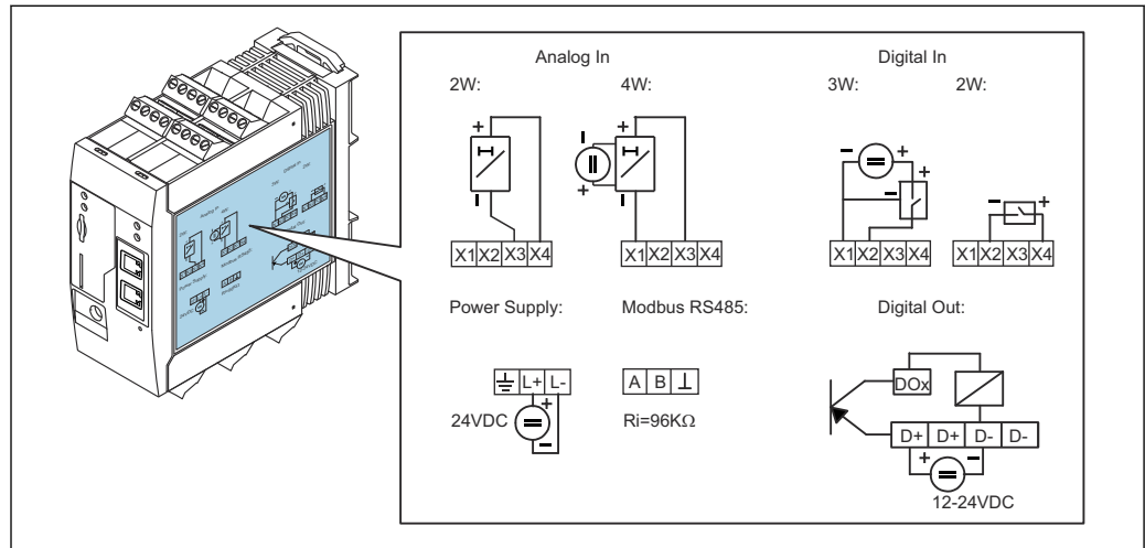
图 8 外壳上的接线端子分配标识
