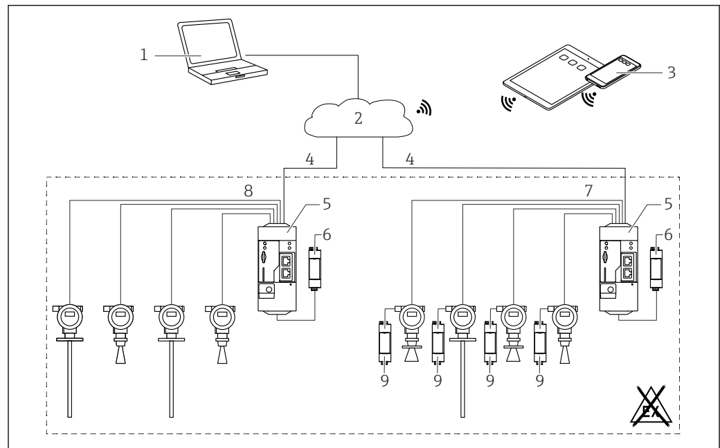
图 3 Fieldgate FXA42 系统架构 (带 4 ... 20 mA 模拟量输入)
