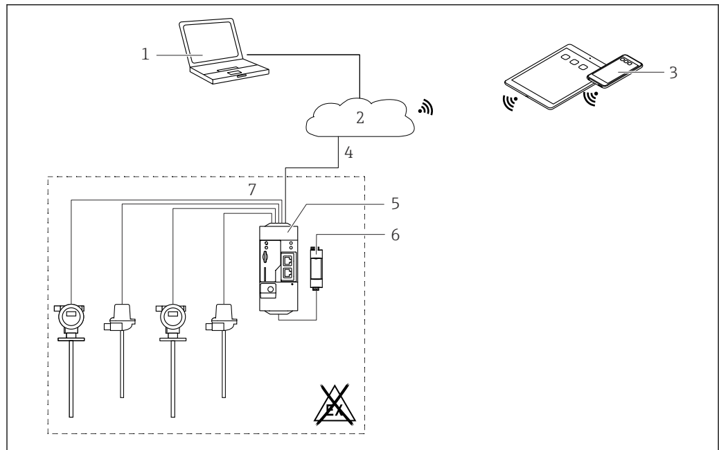
图 4 Fieldgate FXA42 系统架构 (带数字量输入)
