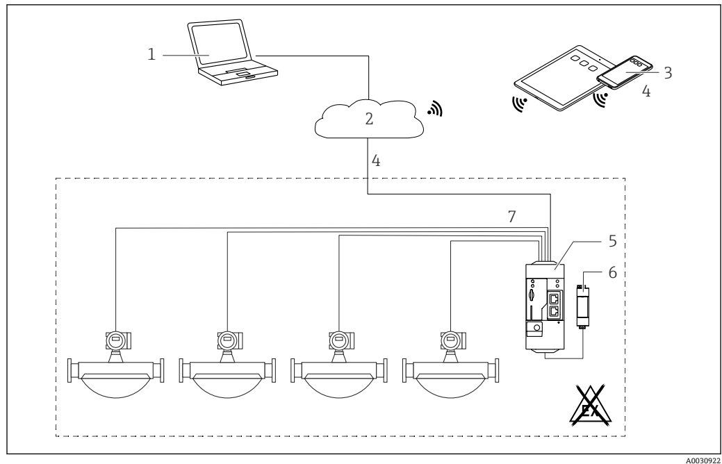
图 5 Fieldgate FXA42 的系统架构 (连接脉冲计数器)
