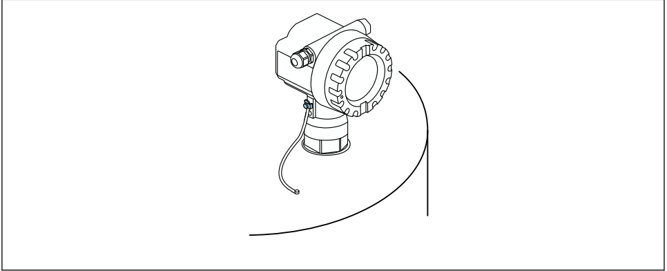
8 Dış topraklama terminali pozisyonu, F12 muhafaza örneği
