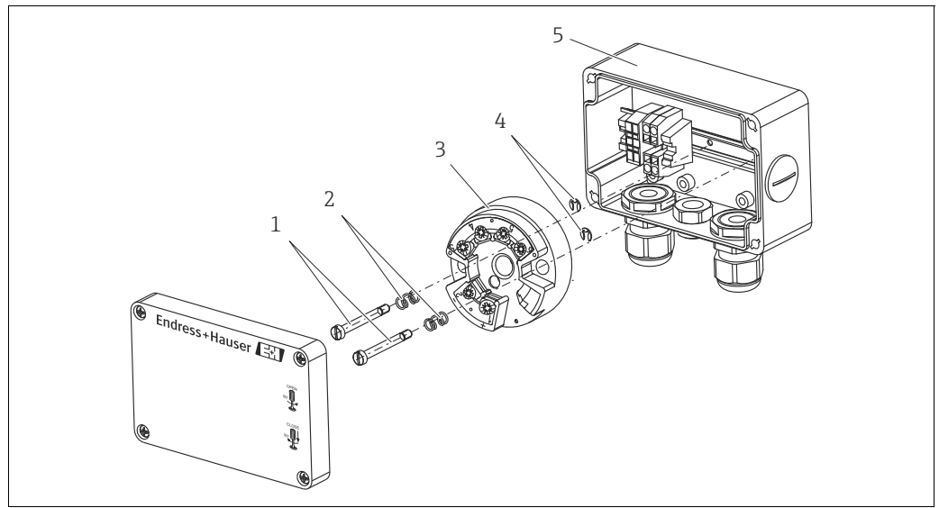
Temperaturkopftransmitter mit Anschlusskasten
