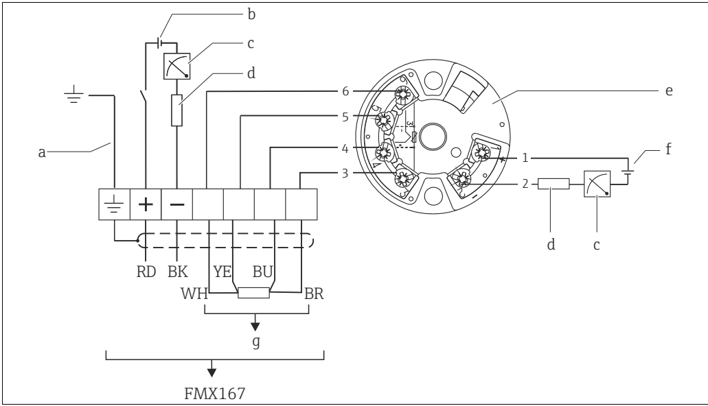
Waterpilot FMX167 mit Pt100 und Temperaturkopftransmitter TMT181 (4...20 mA) 1) ; Variante "5", Merkmal 70 im Bestellcode
