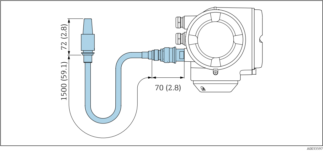
36 Unità mm (in)
