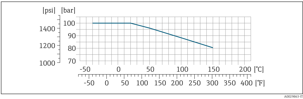
26 Con materiale connessione 1.4404 (316/316L)
