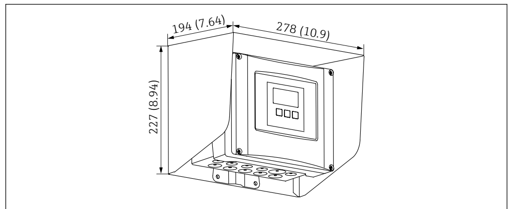
68 Tampa de proteção contra tempo para invólucro de campo de policarbonato. Unidade de medida mm (in)
