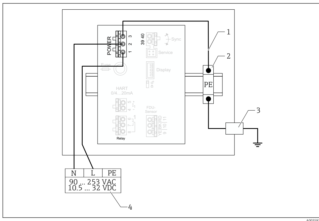
23 Conexão da fonte de alimentação no invólucro de campo de alumínio
