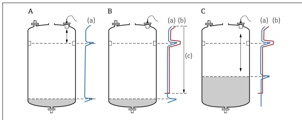
49 Princípio de operação da função de supressão de ecos de interferência (mapeamento)
