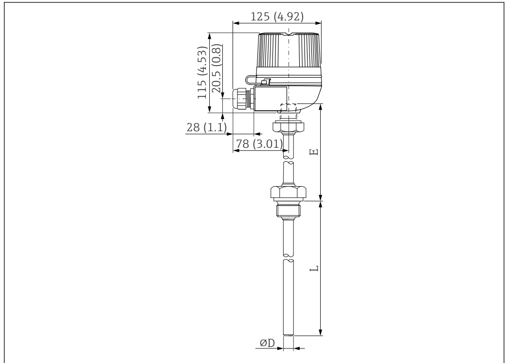
73 Estrutura do Omnigrad S TR61; dimensões: mm (pol.)
