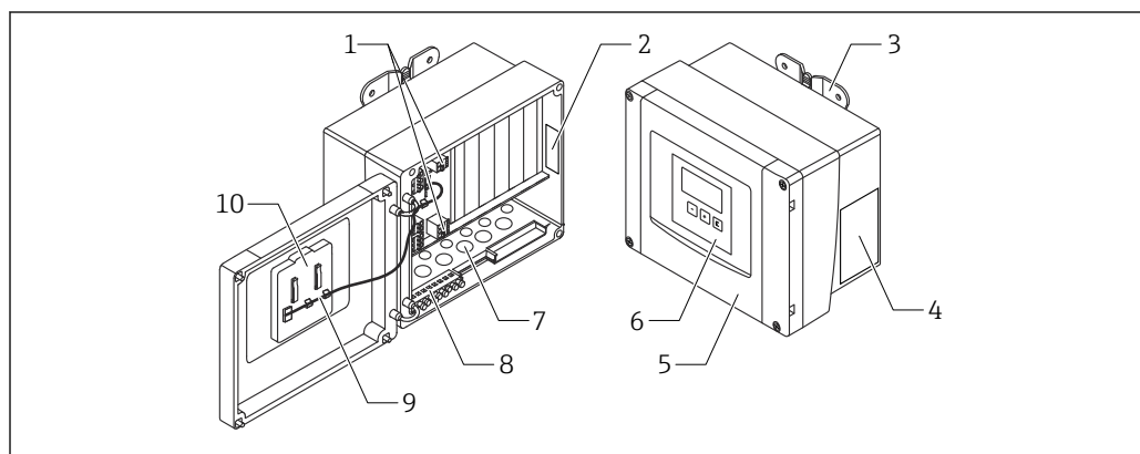
1 Peças do Prosonic S no invólucro de campo de policarbonato
