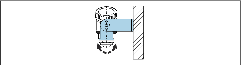
4 설치 브래킷을 사용한 설치, 조정 가능
