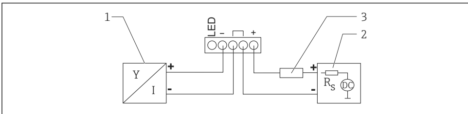
7 HART 계기 및 RIA15 프로세스 디스플레이(조명 없음) 기능도
