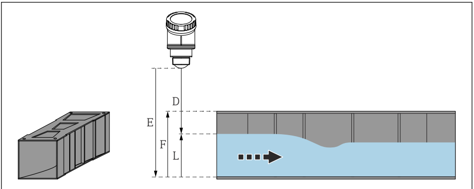
17 예: 가파기(Khafagi) 벤추리 수로
