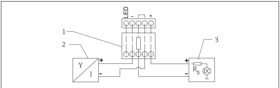
☐ 9 HART 계기 기능도, RIA15(조명 없음), HART 통신 저항 모듈
