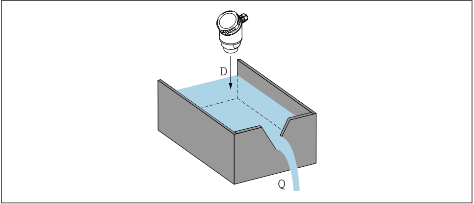
16 액체 유량 측정을 위한 구성 파라미터
