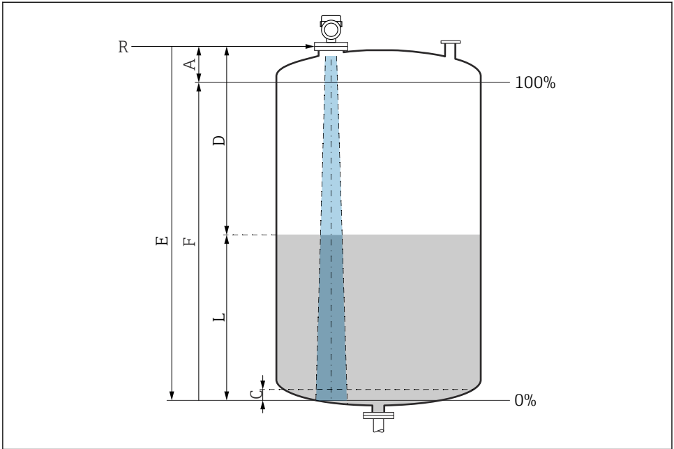
☞ 14 액체 레벨 측정 설정 파라미터
