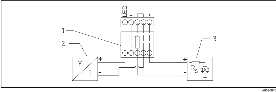
☐ 10 HART 계기 기능도, RIA15(조명 있음), HART 통신 저항 모듈
