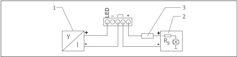
☐ 8 HART 계기 및 RIA15 프로세스 디스플레이(조명 있음) 기능도
