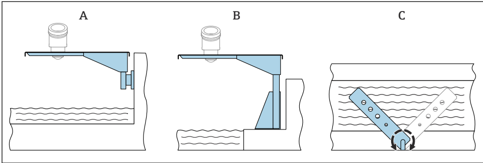
■ 5 캔틸레버 설치, 피벗
