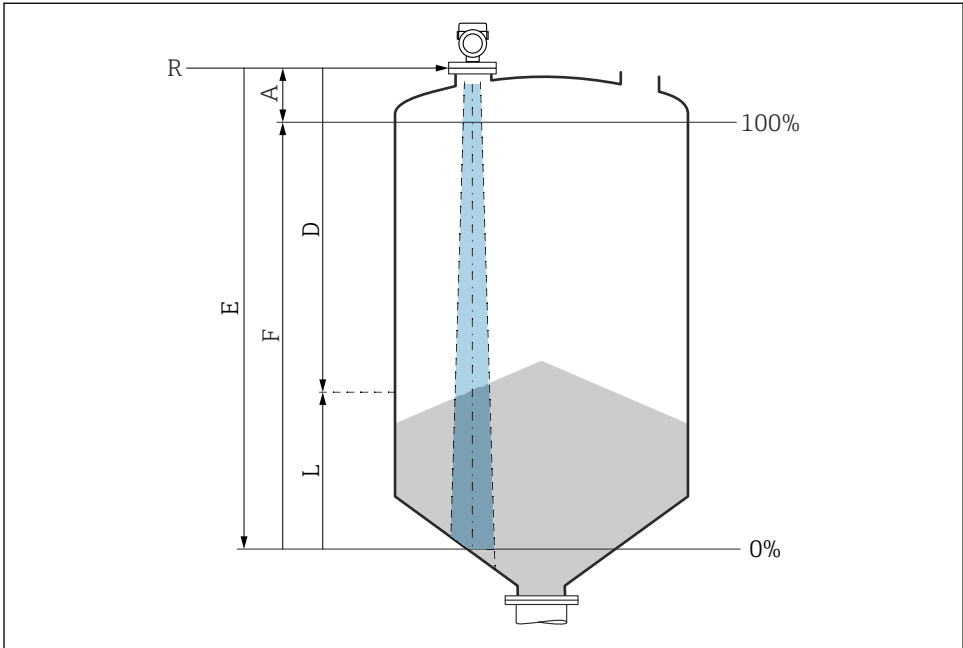
15 본체 레벨 측정 구성 파라미터
