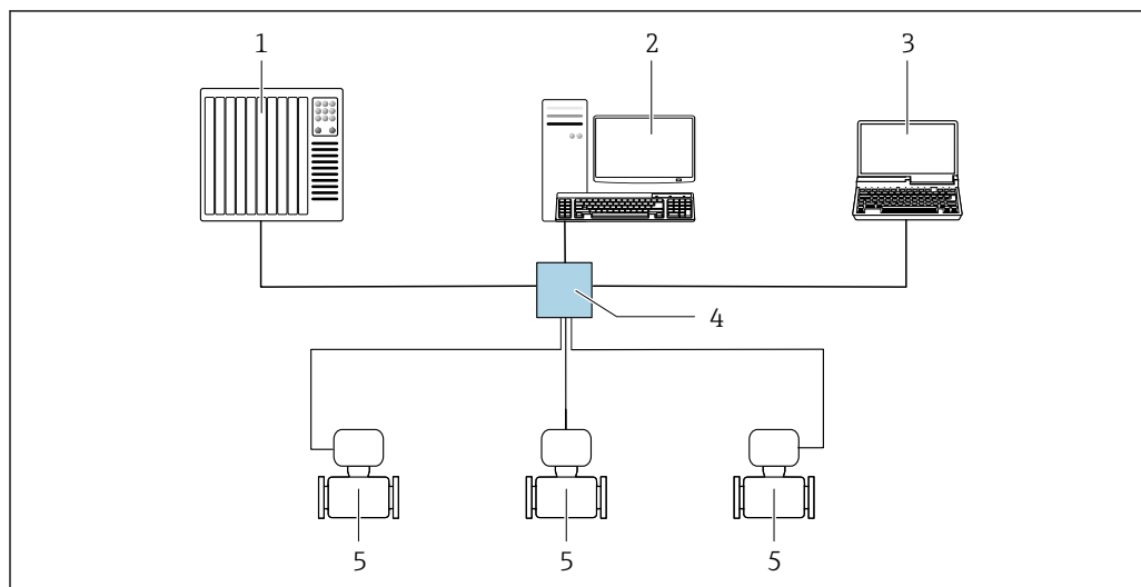
図 44 Modbus TCP over Ethernet - 100 Mbit/s 経由のリモート操作用オプション：スター型トポロジー
