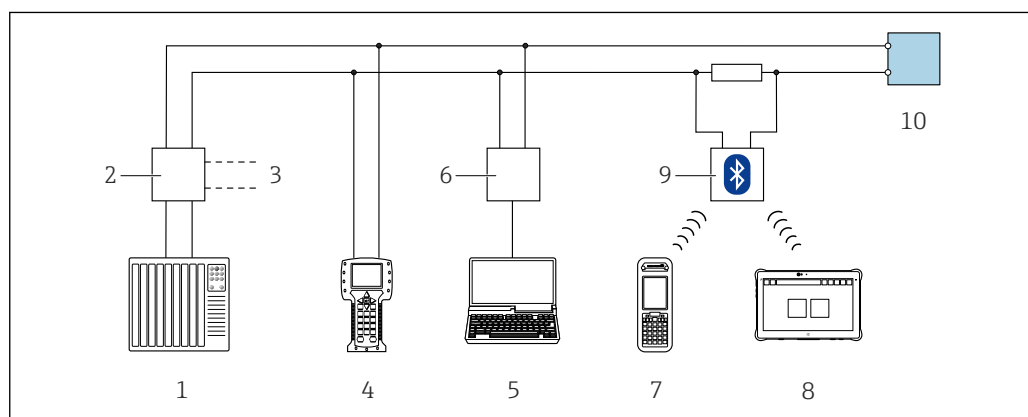
図 38 HART プロトコル経由のリモート操作オプション (パッシブ)
