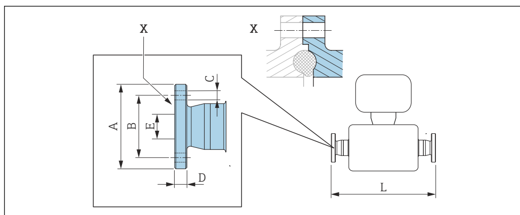
図 25 Xの詳細：非対称型プロセス接続；着色部分が供給されます。
