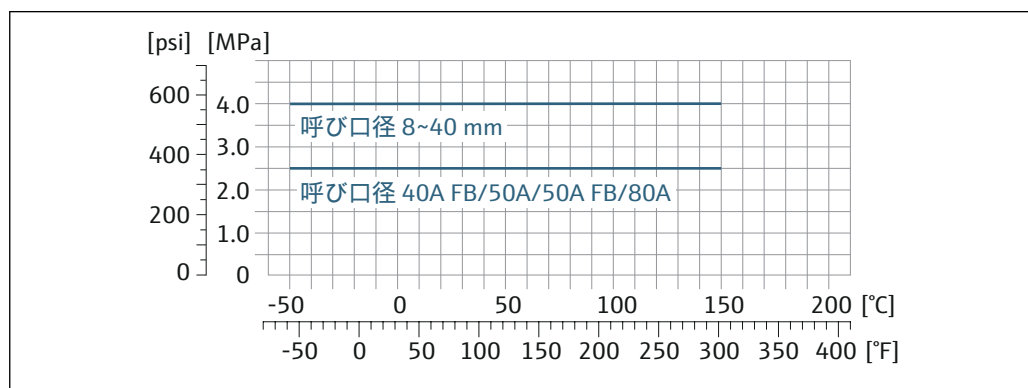
図 21 接続部材質 グレード 2 チタン
