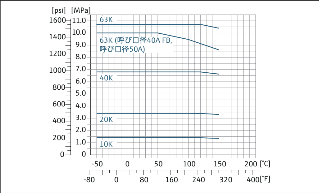
図 18 フランジ材質 1.4301 (SUS 304 相当)。接液部：チタン
