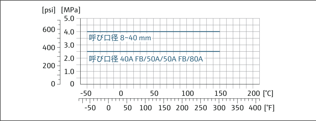
図 20 接続部材質 グレード 2 チタン
