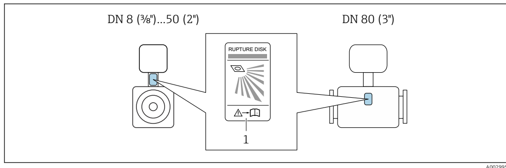
1 Autocollant du disque de rupture
