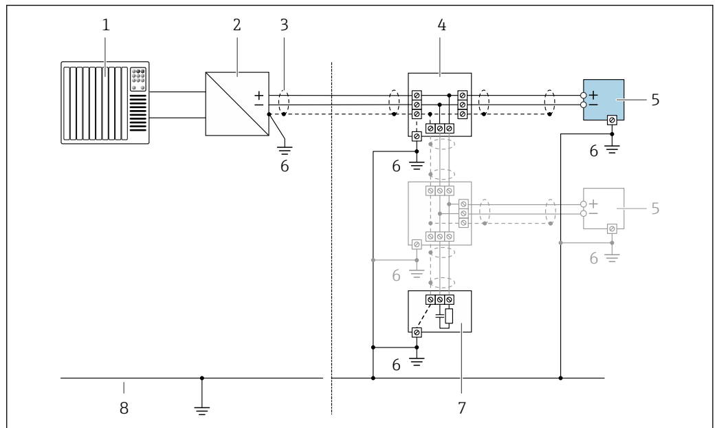
20 Exemple de raccordement pour FOUNDATION Fieldbus
