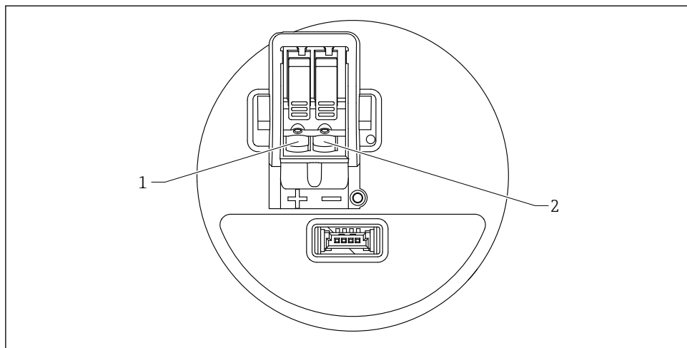
11 Esquema de ligação elétrica
