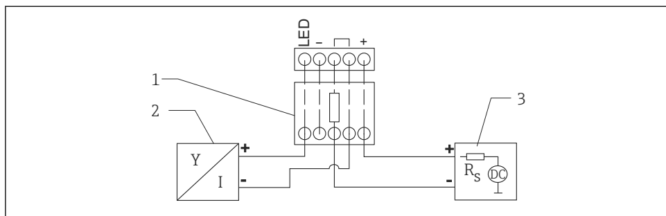
10 Diagrama de função do equipamento HART, RIA15 com iluminação, módulo de resistor de comunicação HART
