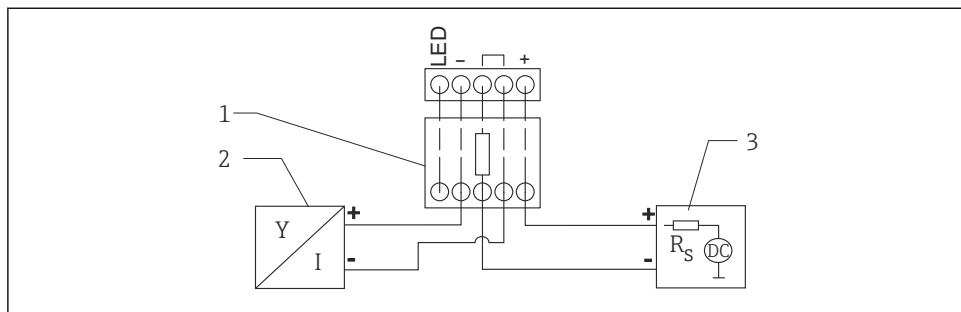
9 Diagrama de função do equipamento HART, RIA15 sem iluminação, módulo de resistor de comunicação HART
