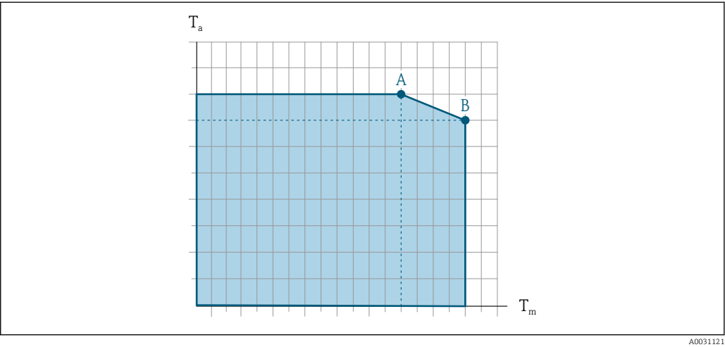
35 Rappresentazione esemplificativa, valori nella tabella sottostante. T_a Temperatura ambiente T_m Temperatura del fluido A Temperatura del fluido massima consentita T_m con T_{a\,max} = 60\,^{\circ}\text{C} (140 °F); temperature del fluido superiori T_m richiedono una temperatura ambiente ridotta T_a B Temperatura ambiente massima consentita T_a per la temperatura del fluido massima specificata T_m del sensore
