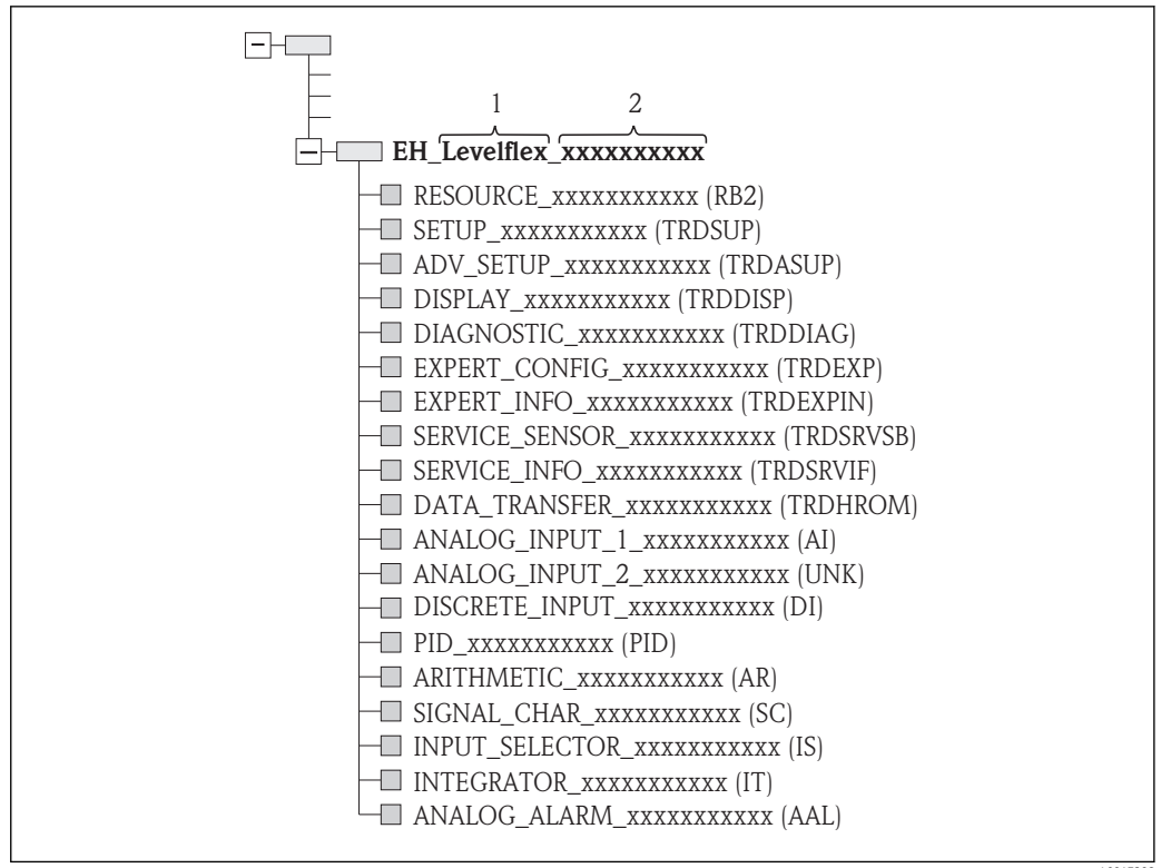
13 Représentation typique dans un logiciel de configuration après l'établissement de la connexion
