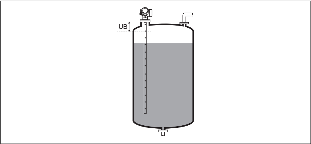
30 Distance de blocage (UB) pour la mesure dans les liquides
