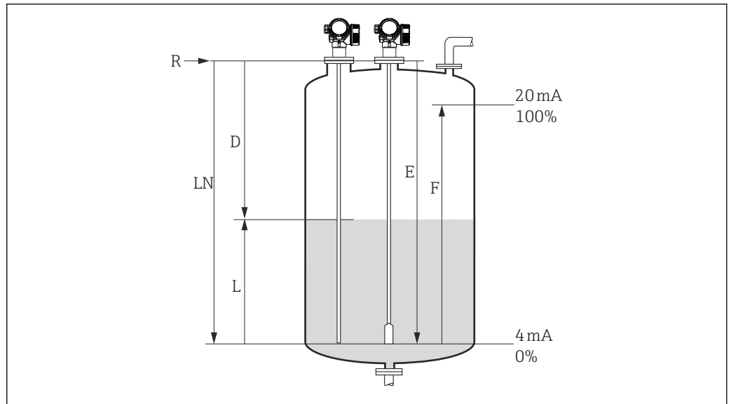
16 Paramètres de configuration pour la mesure de niveau dans les liquides
