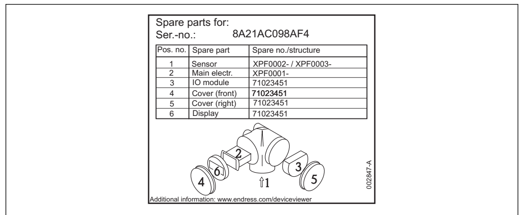
23 Exemple de plaque signalétique dans le couvercle du compartiment de raccordement
