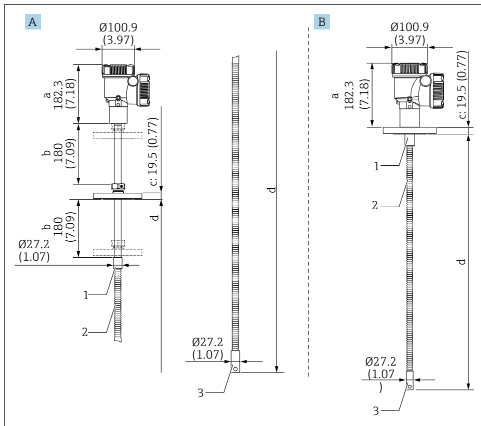
6 Przetwornik + sonda do pomiaru temperatury średniej. Jednostka miary mm (in)
