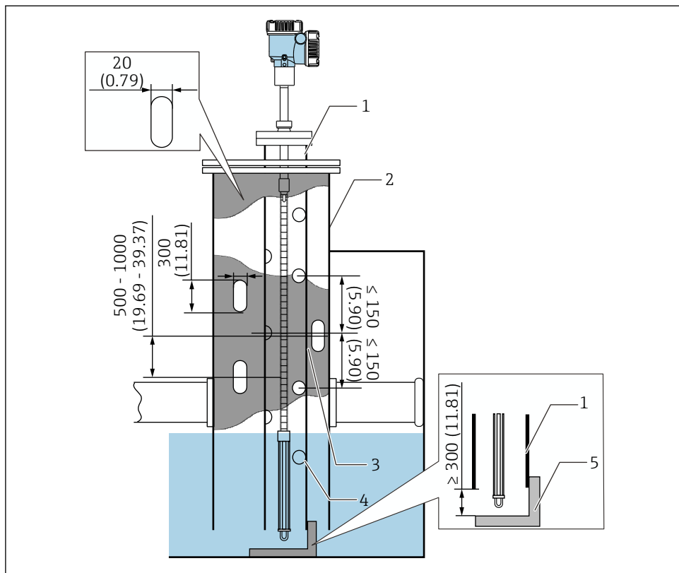
30 Zastosowanie rury osłonowej. Jednostka miary mm (in)
