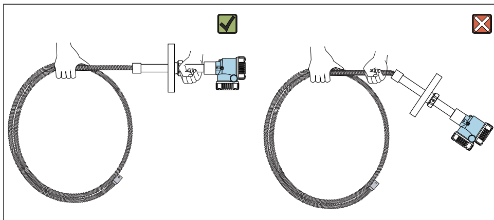
15 Rozpakowanie sondy NMT81
