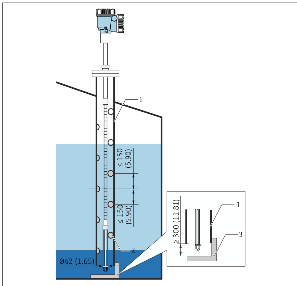
27 Rura osłonowa. Jednostka miary mm (in)
