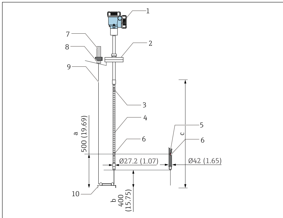
▣ 24 Zastosowanie górnego zaczepu. Jednostka miary mm (in)
