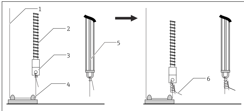
25 Montaż z zastosowaniem górnego zaczepu, rys. 1
