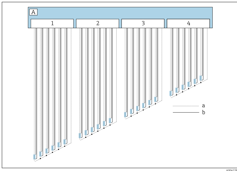
35 Schemat podłączenia czteroprzewodowego
