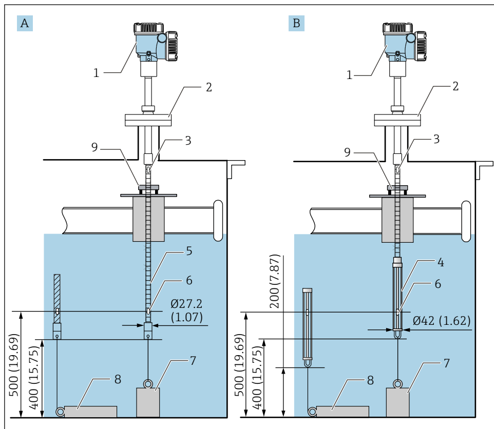
31 Zastosowanie ucha prowadzącego i obciążnika kotwicowego. Jednostka miary mm (in)
