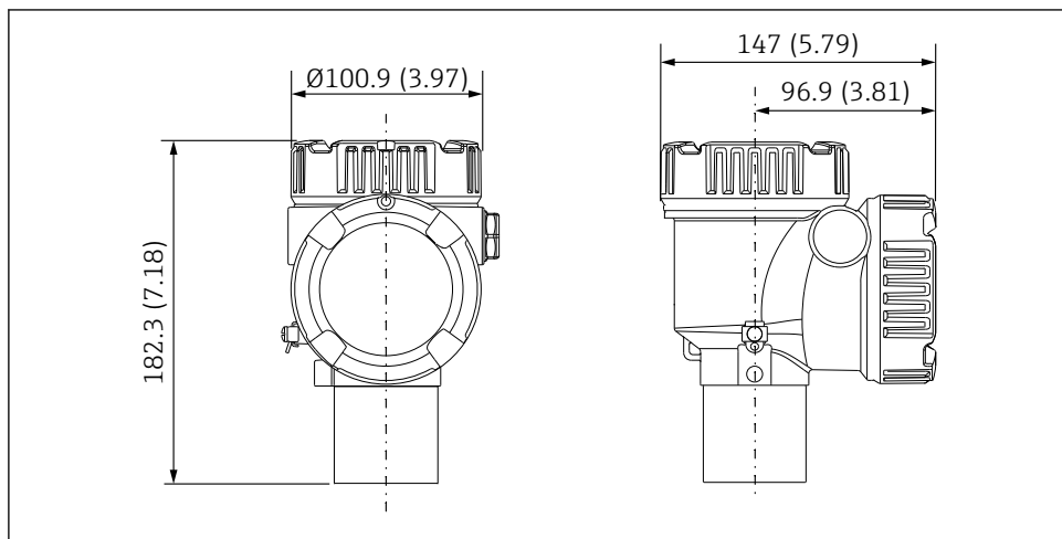
3 Przetwornik standardowy. Jednostka miary mm (in)
