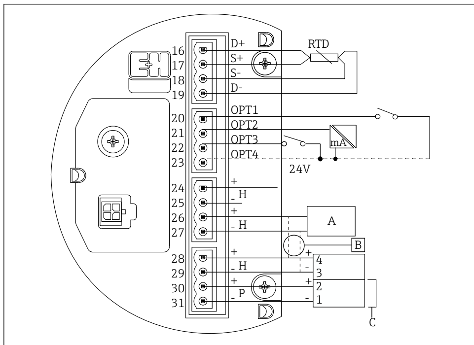
38 Zaciski (iskrobezpieczne) koncentratora NRF590
