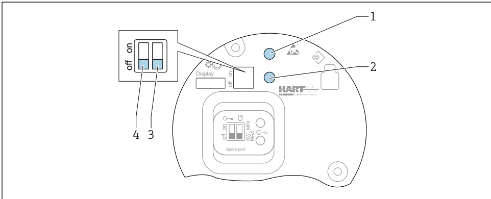
15 HART 기판의 작동 키 및 DIP 스위치
