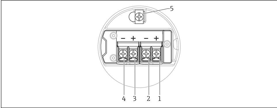
10 연결부 단자 할당, 4~20 mA HART + 4~20 mA 아날로그, 이중 격벽 하우징
