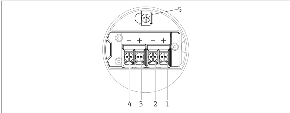
11 연결부 단자 할당, 4~20 mA HART, 스위칭 출력, 이중 격벽 하우징
