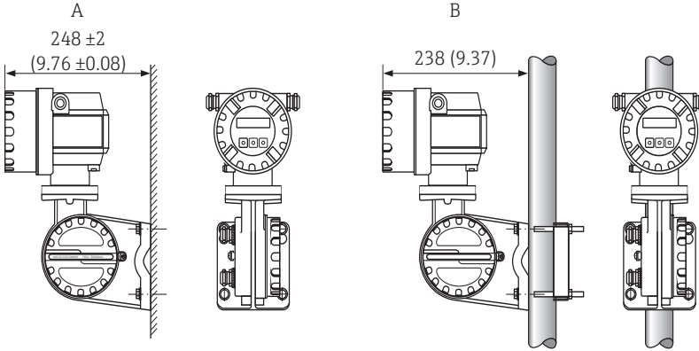
Fig. 1: Montaje del transmisor (versión separada)
