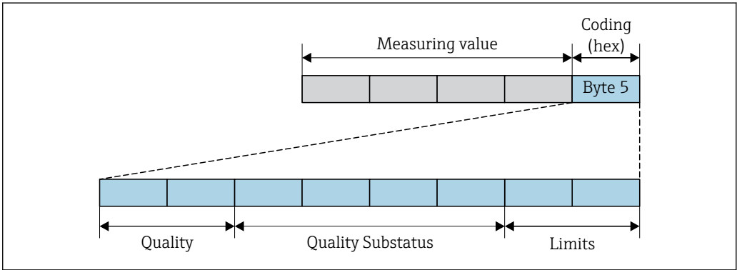
29 Структура байта состояния
